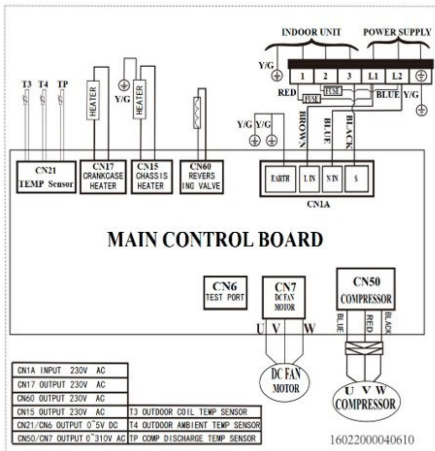
Fig. 6 – 9K - 12K - 18K
