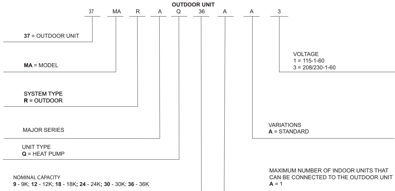
Fig. 1 —Nomenclature
