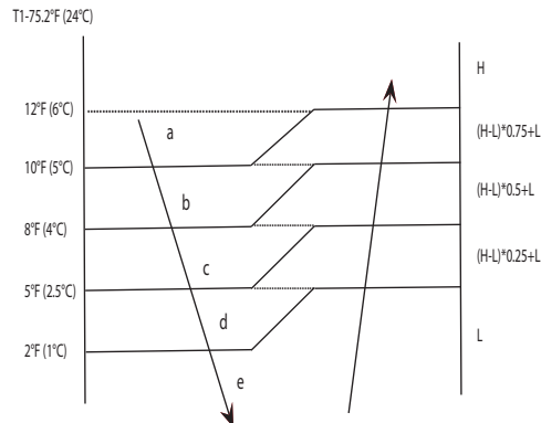
Fig. 13 —AUTO FAN Mode
