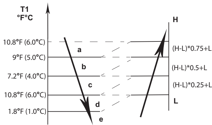
Fig. 16 —AUTO FAN Running Rules
