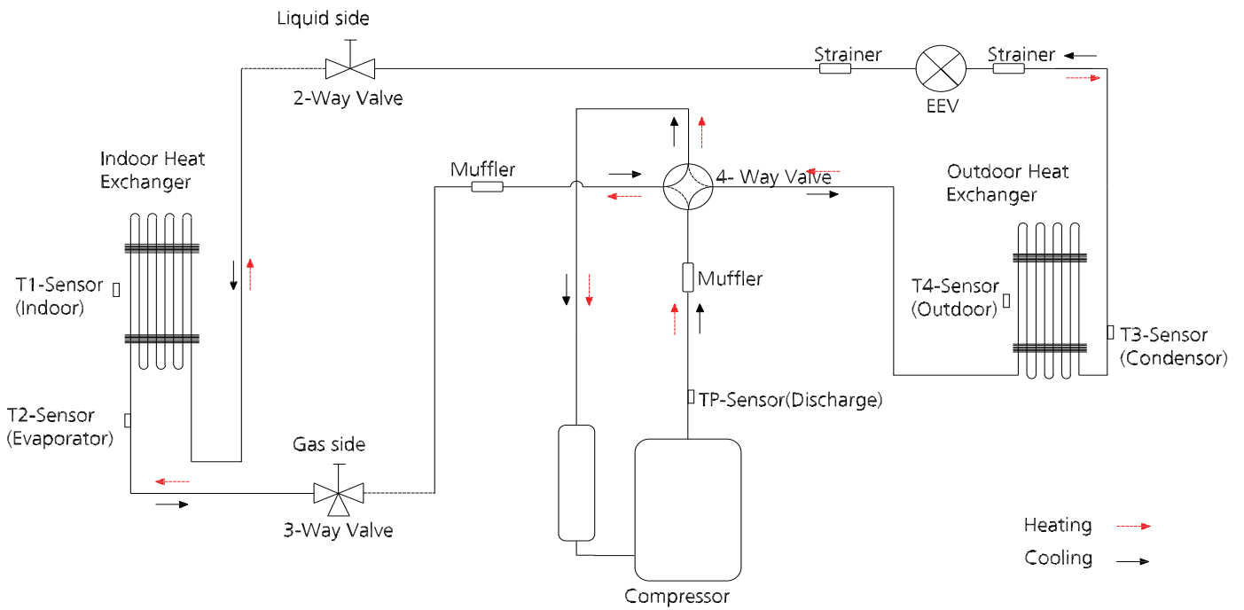
Fig. 6 —Sizes 6K - 12K
