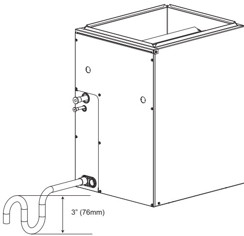
Fig. 8 - Condensate Trap
