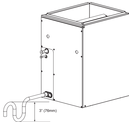
Fig. 8 - Condensate Trap
