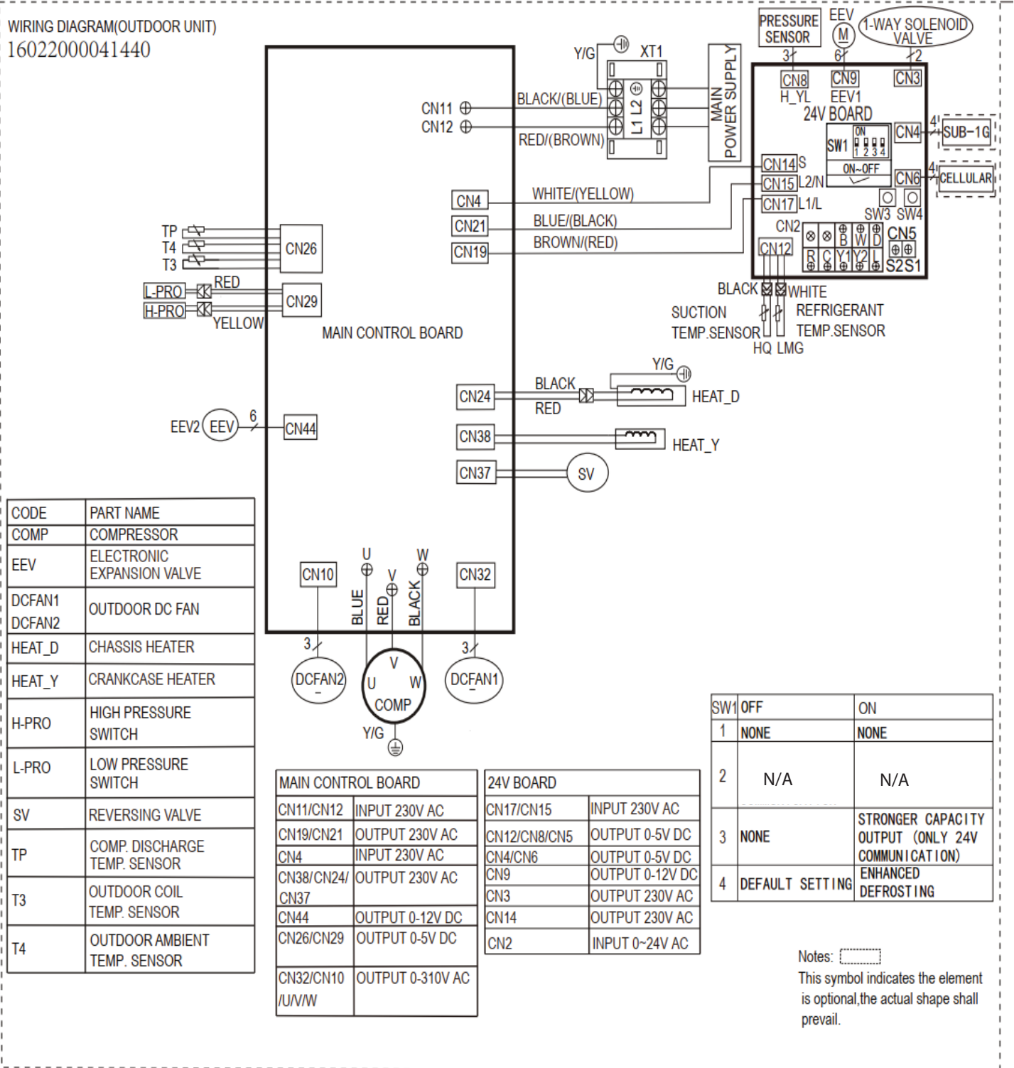
Fig. 29 — Size 60K
