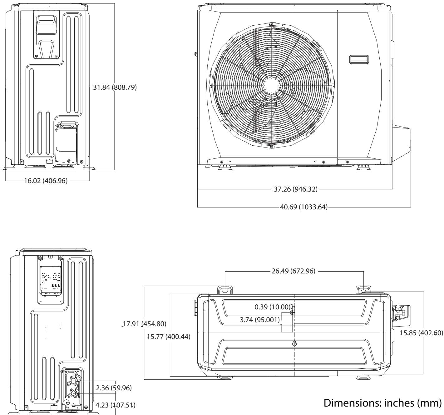
Fig. 5 —Size 30K
