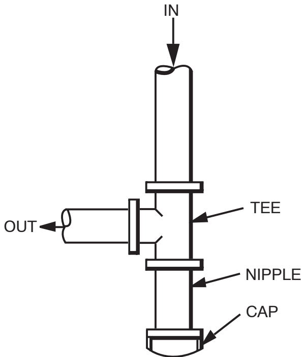
Fig. 9 - Sediment Trap
