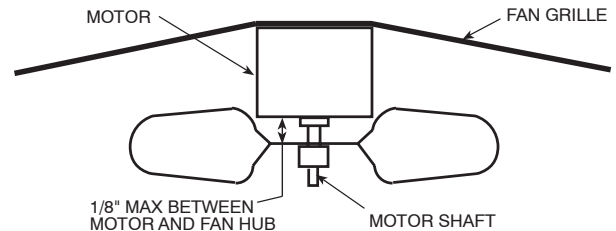
Fig. 16 - Fan Blade Clearance
