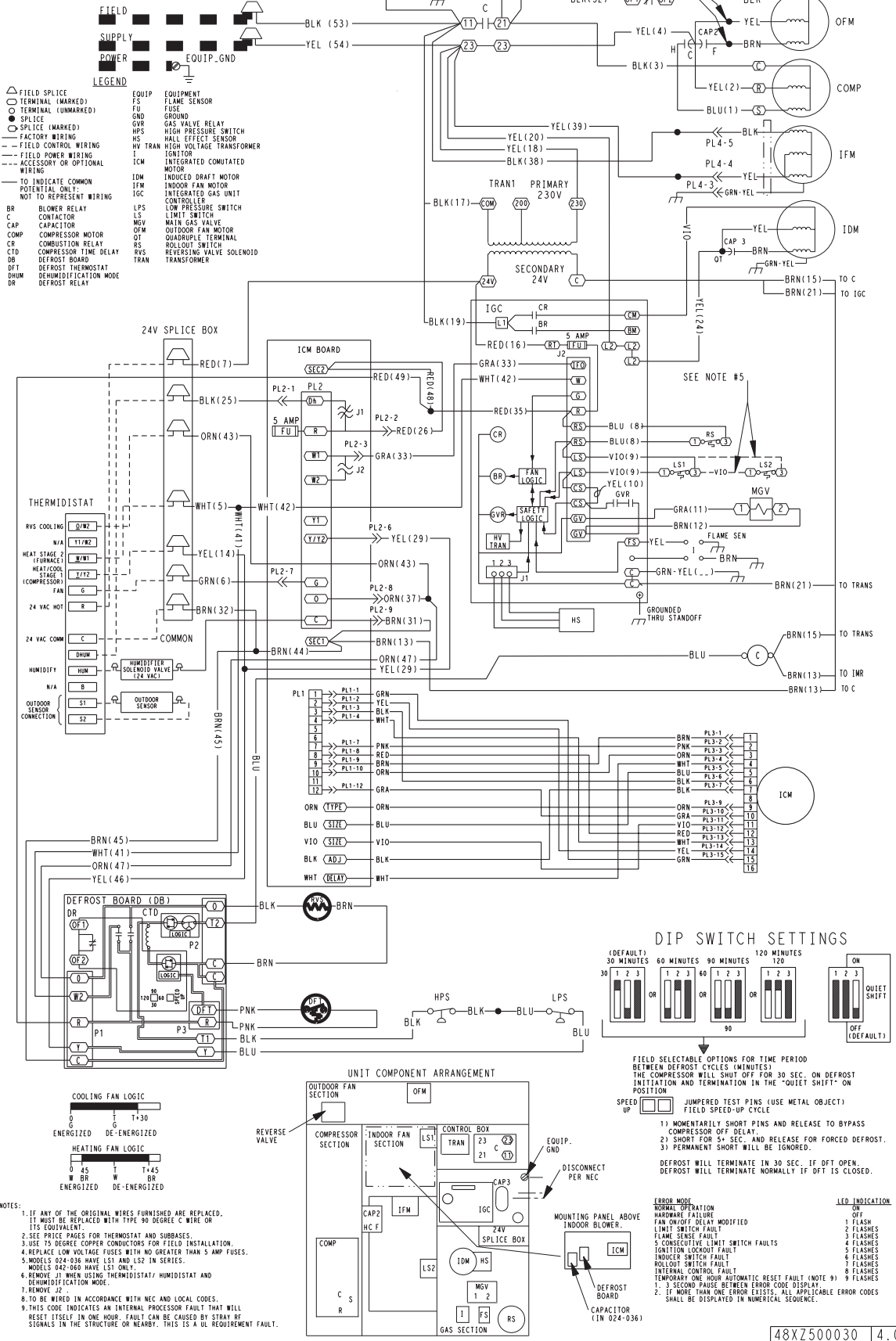
Fig. 19 - 208/230-1-60 Wiring Diagram, Unit 48XZ
