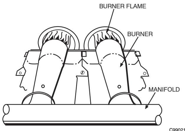
Fig. 18 - Monoport Burner
