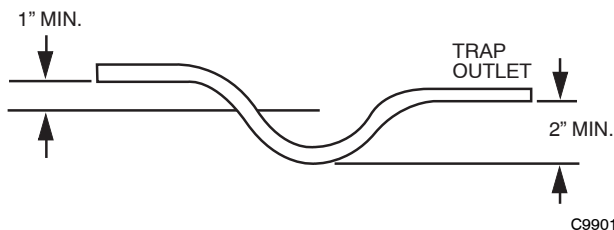
Fig. 8 - Condensate Trap
