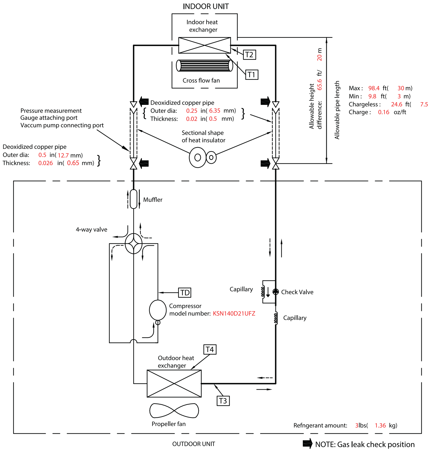
Fig. 9 —18K (208-230V)
