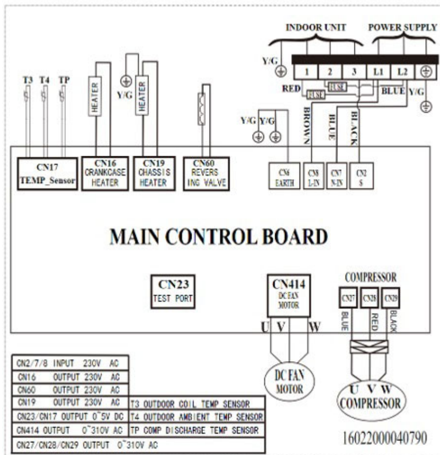
Fig. 7 – 24K (208V/230V)
