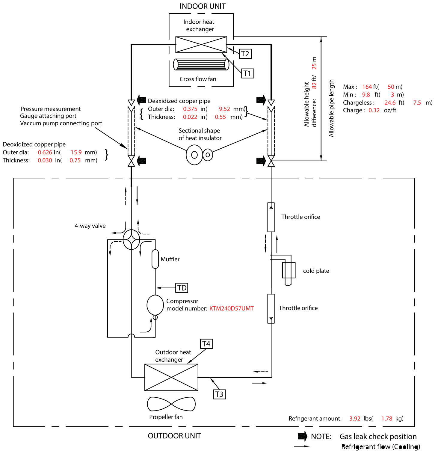
Fig. 10 —24K (208-230V)
