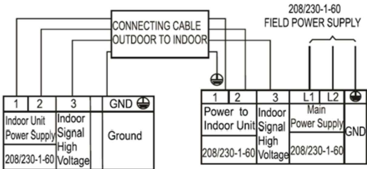
Fig. 4 —9K - 24K (208V/230V)
