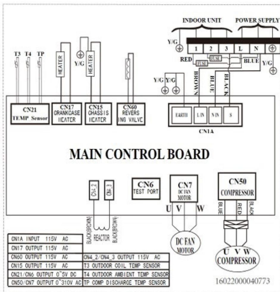
Fig. 5 – 9K - 12K (115V)
