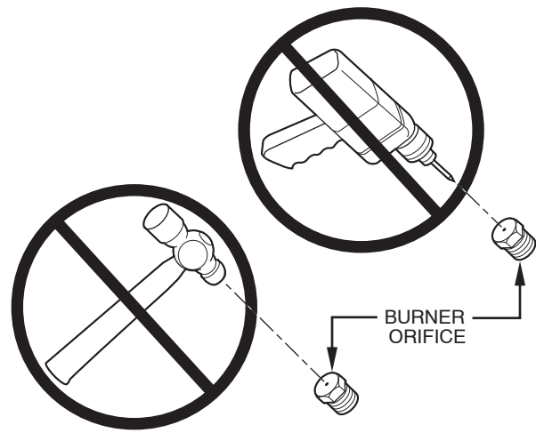
Fig. 54 - Orifice Hole
