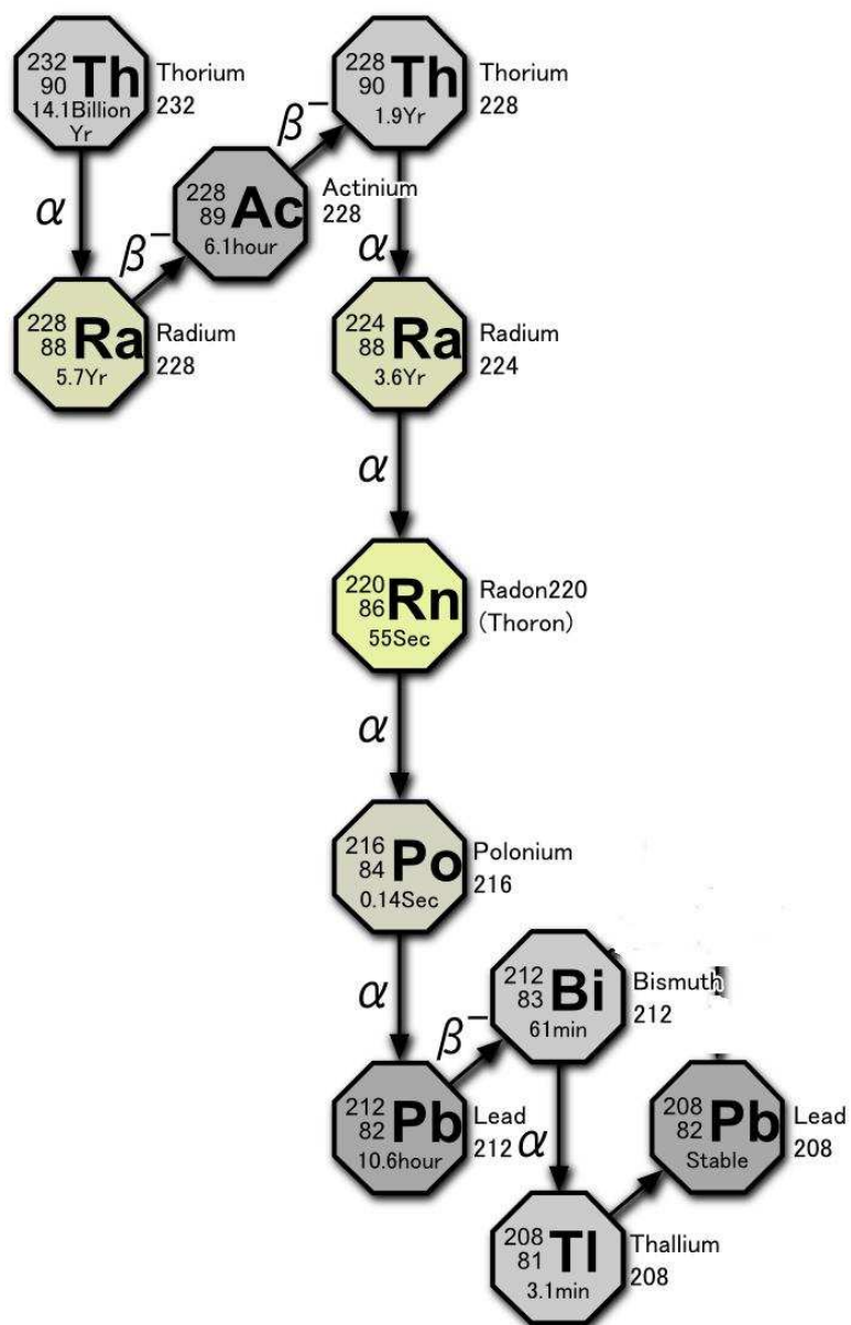
Figura 2.4: Série do Tório com meias-vidas mais longas.
