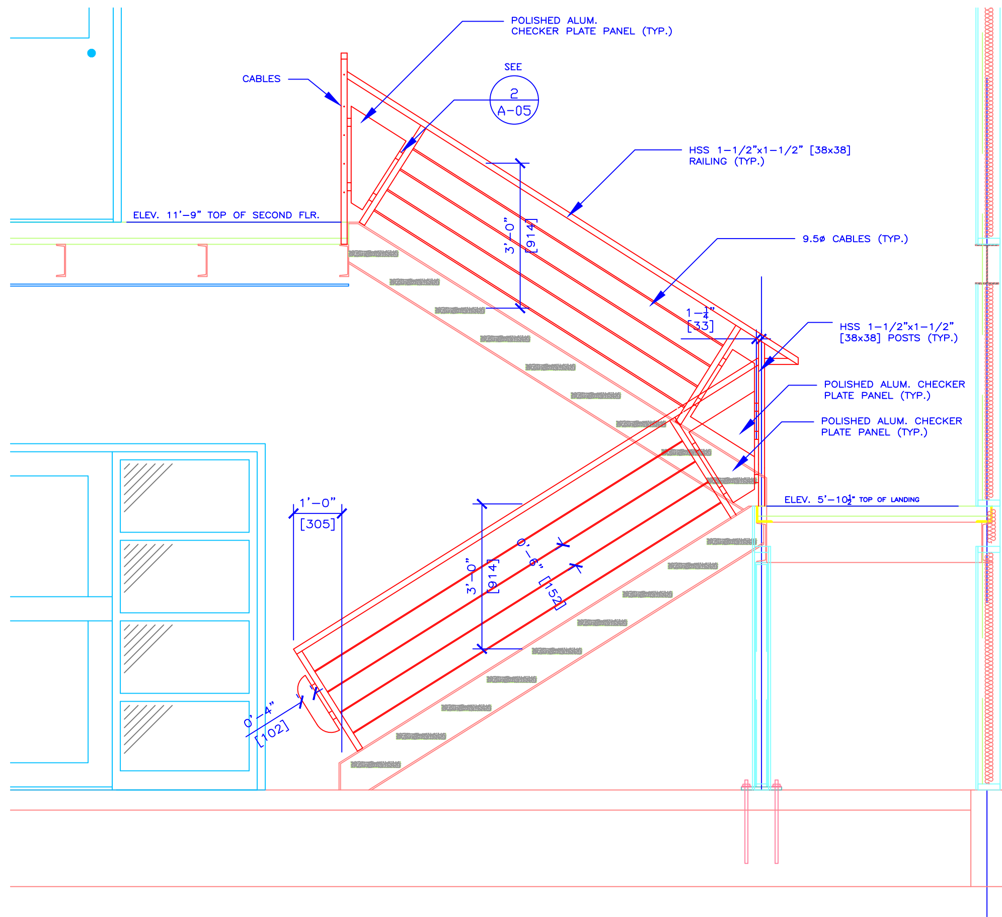
1 STAIR DETAIL 1 Scale: 1/2" = 1'-0"
