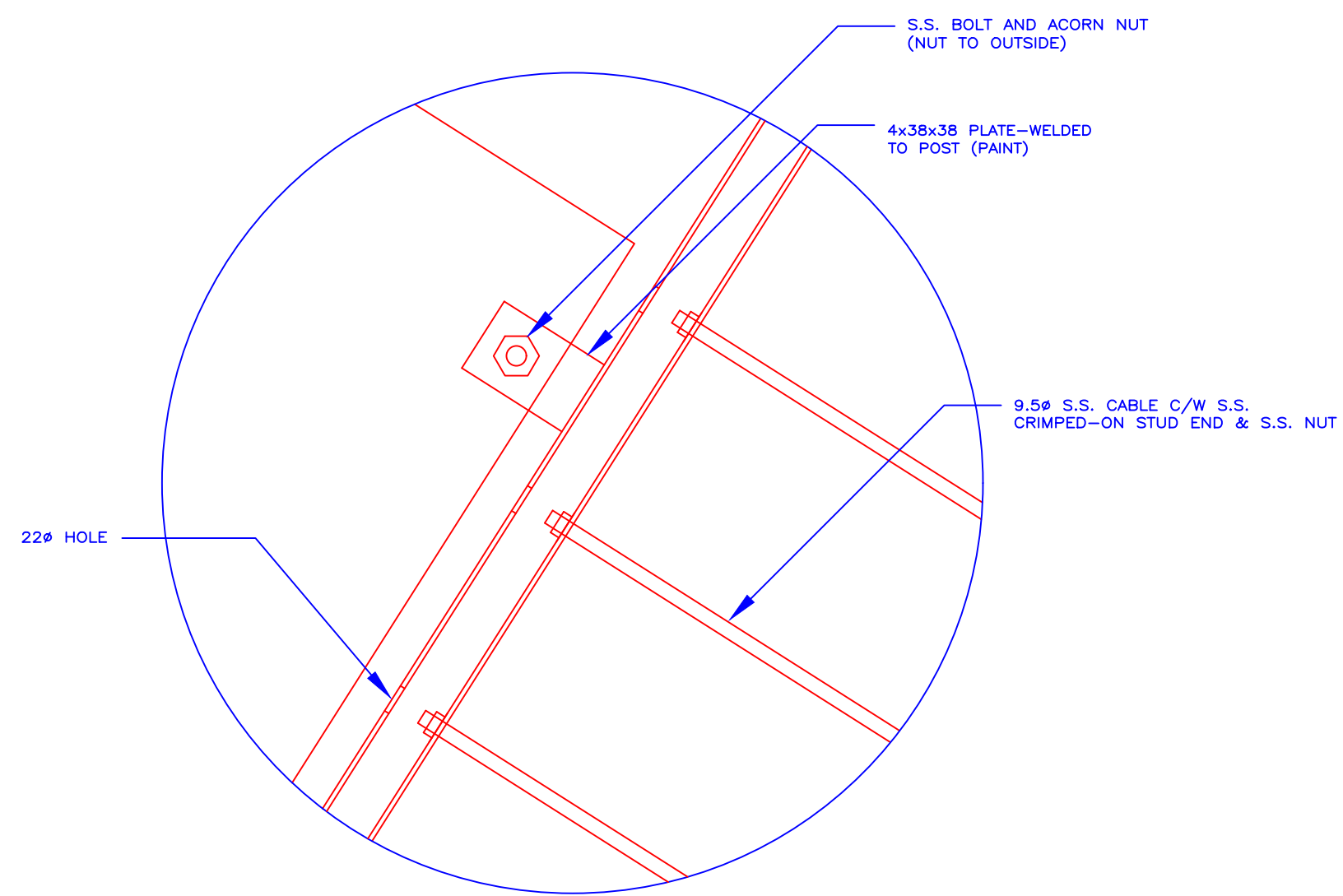
2 STAIR DETAIL 2 Scale: 3" = 1'-0"
