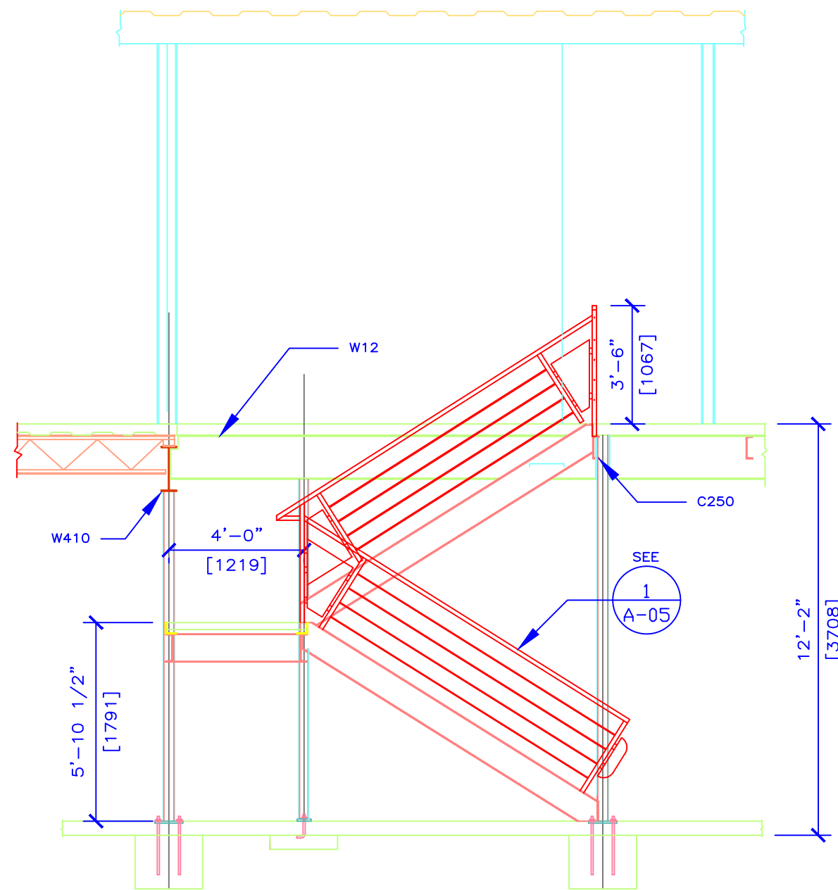
2 STAIR SECTION 2 Scale: 1/4" = 1'-0"
