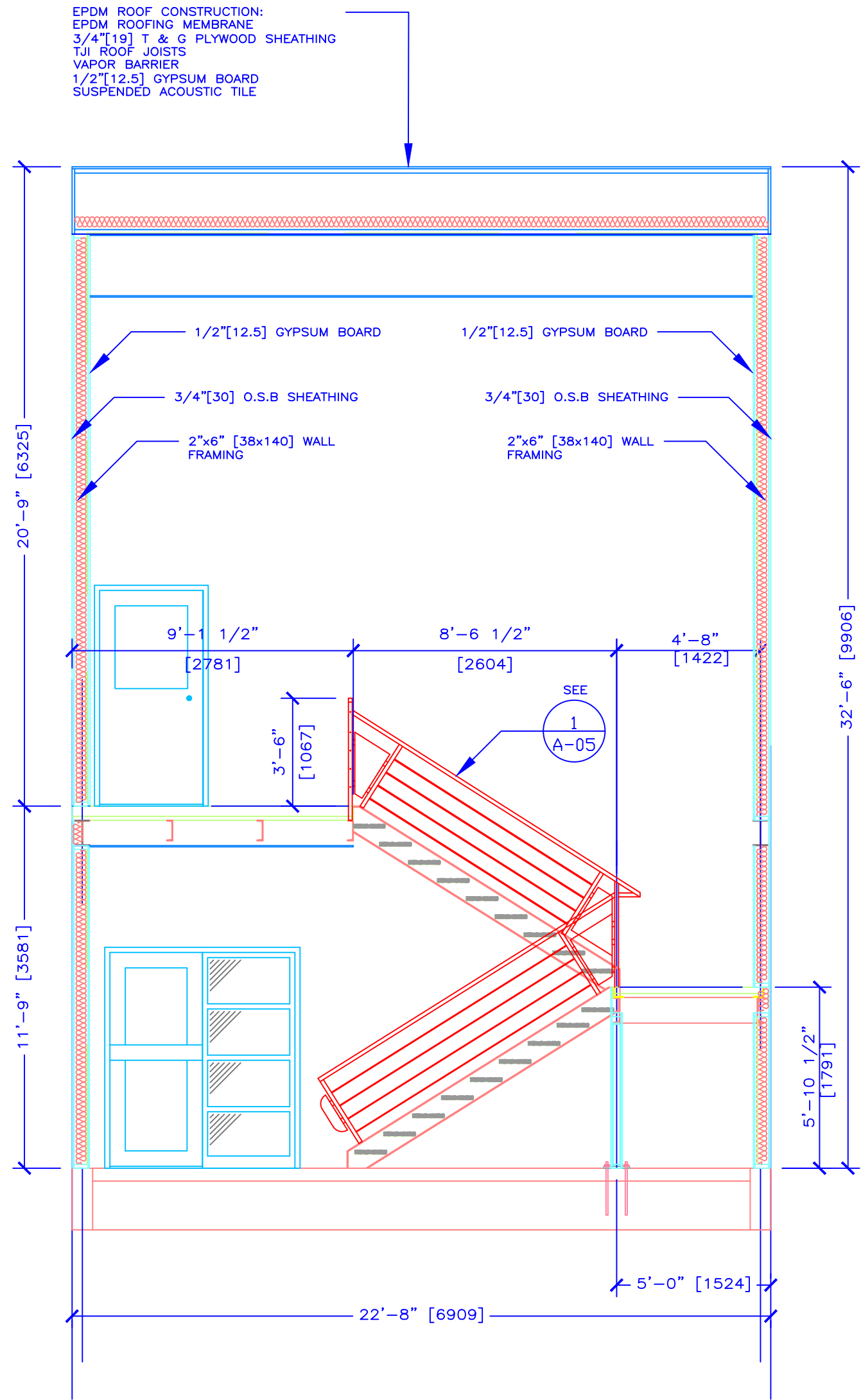
1 STAIR SECTION 1 Scale: 1/4" = 1'-0"
