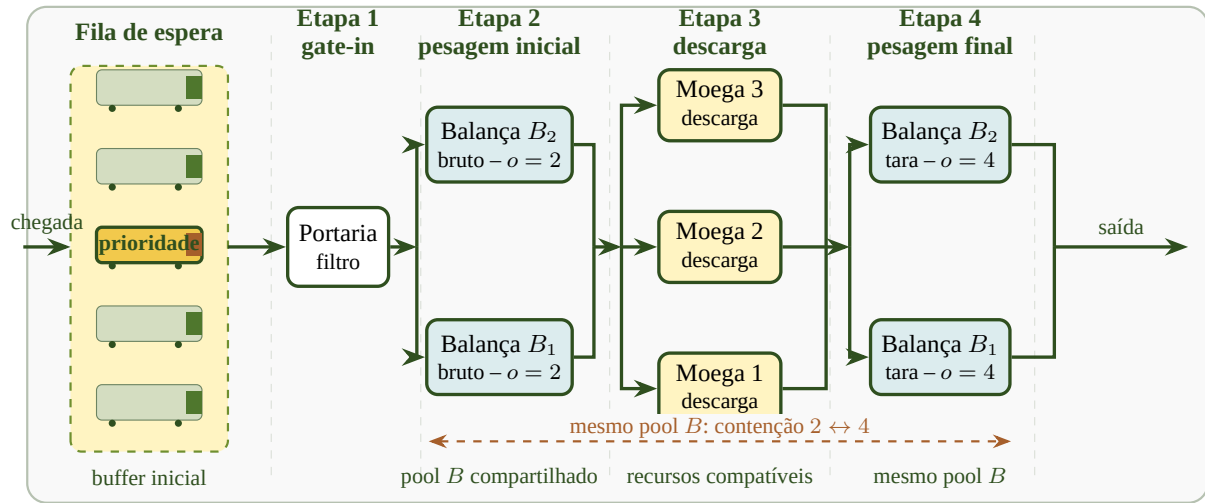
Figura 3 – Leiaute esquemático do pátio de recebimento de grãos (vista superior), com quatro etapas operacionais e balanças físicas compartilhadas. Etapa 1: gate-in (portaria). Etapa 2: peso bruto no pool B de balanças. Etapa 3: descarga (moegas). Etapa 4: tara no mesmo pool B . As setas tracejadas indicam a contenção reentrante entre as etapas 2 e 4; caminhões com prioridade mandatória estão destacados em amarelo-pequi.
