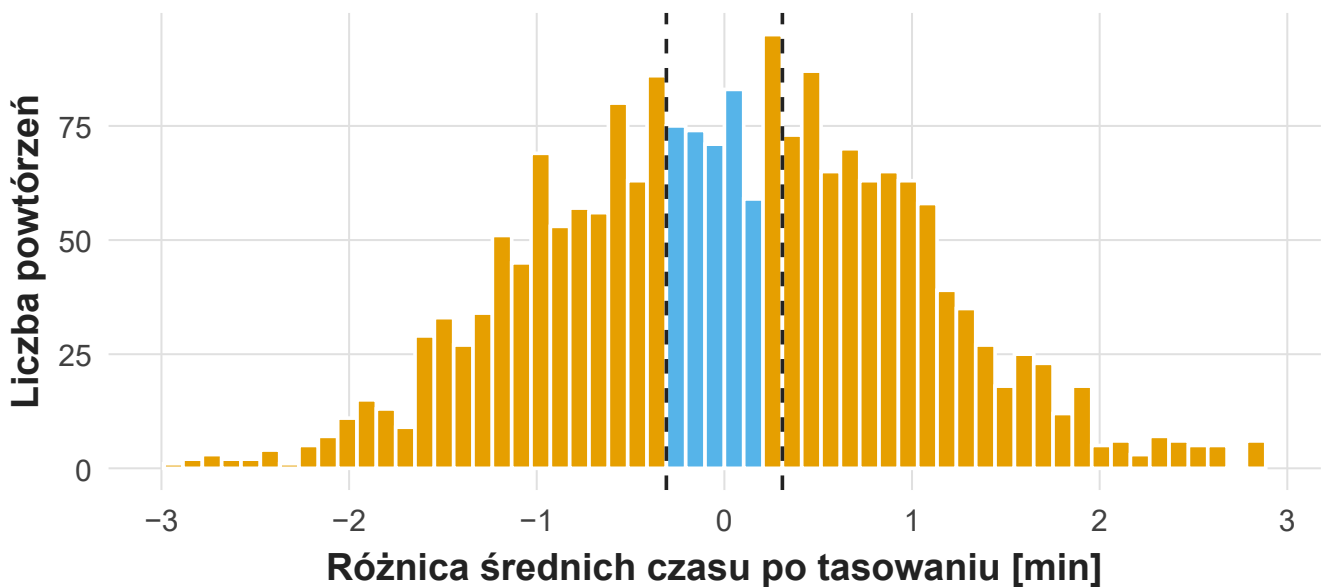
Rysunek 8: Rozkład zerowy tasowania etykiet dla czasu: histogram 1999 różnic średnich po przestawieniu etykiet. Oś pozioma: różnica w minutach; oś pionowa: liczba powtórzeń. Histogram leży od -2,98 do 2,85 minuty wokół zera; linie przerywane przy -0,309 i 0,309 obejmują wąski środek, a wyróżnione słupki na liniach i poza nimi zawierają 1544 powtórzenia.
