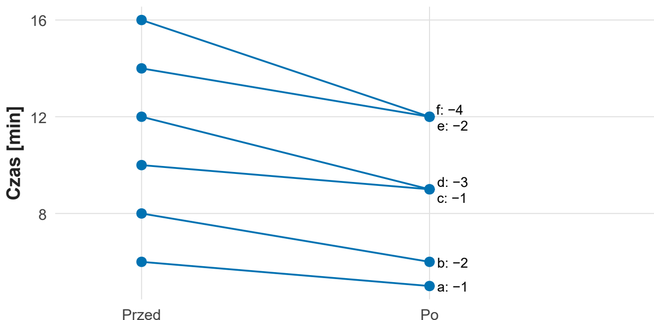
Rysunek 12: Sześć par: czas przed instruktażem i po nim. Oś pionowa: czas w minutach. Każdy odcinek łączy dwa pomiary jednej osoby; wszystkie sześć odcinków opada, o 1 do 4 minut, a etykiety przy pomiarze po podają osobę i zmianę.
