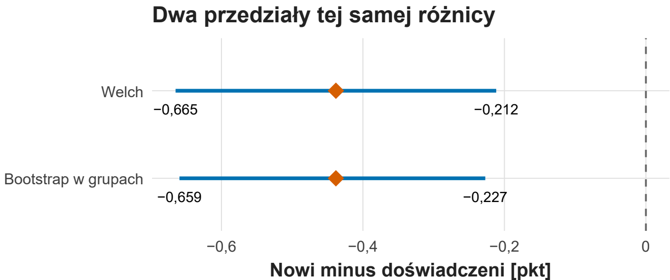
Rysunek 5: Dwa przedziały tej samej różnicy nowi minus doświadczeni. Oś pozioma: różnica w punktach. Welch: od -0,665 do -0,212 ; bootstrap w grupach: od -0,659 do -0,227 ; romby przy -0,438 ; linia przerywana zera leży na prawo od obu odcinków.
