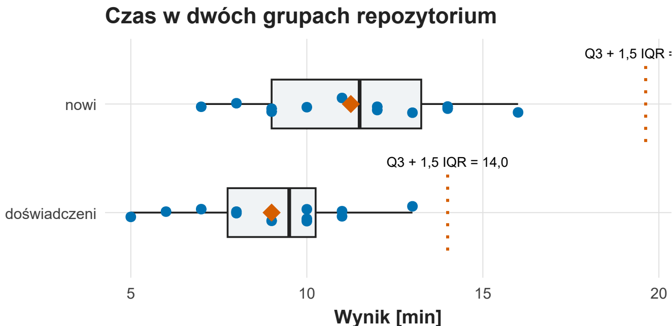
Rysunek 9: Czas w dwóch grupach repozytorium. Oś pozioma: czas w minutach; punkty: czasy wszystkich osób; pudełko: kwartyle i mediana; romb: średnia grupy; linia kropkowana: granica Q3 + 1,5 \text{ IQR} .
