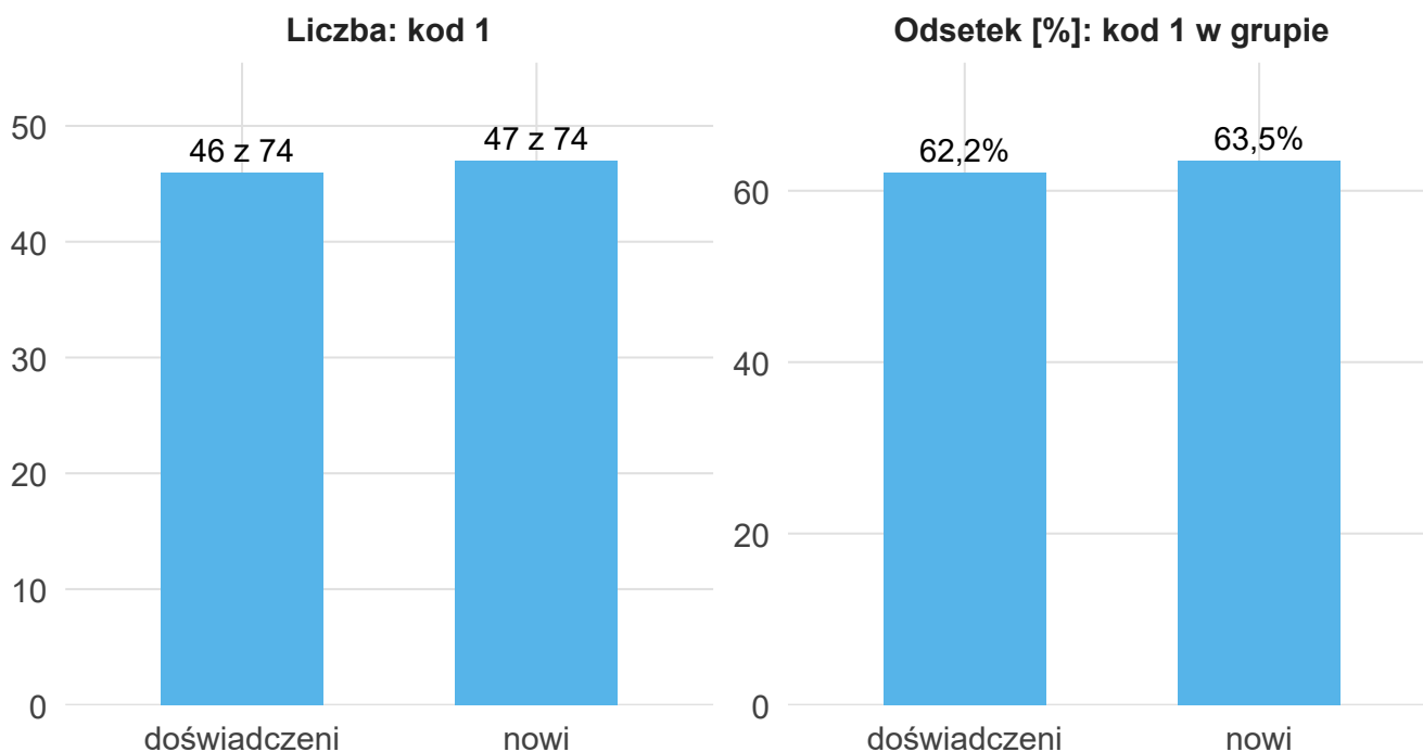
Rysunek 8: Druga analiza własnego wariantu: kod 1 w grupach (liczba i odsetek) albo kompletne pary indeksu i drugiej zmiennej.
