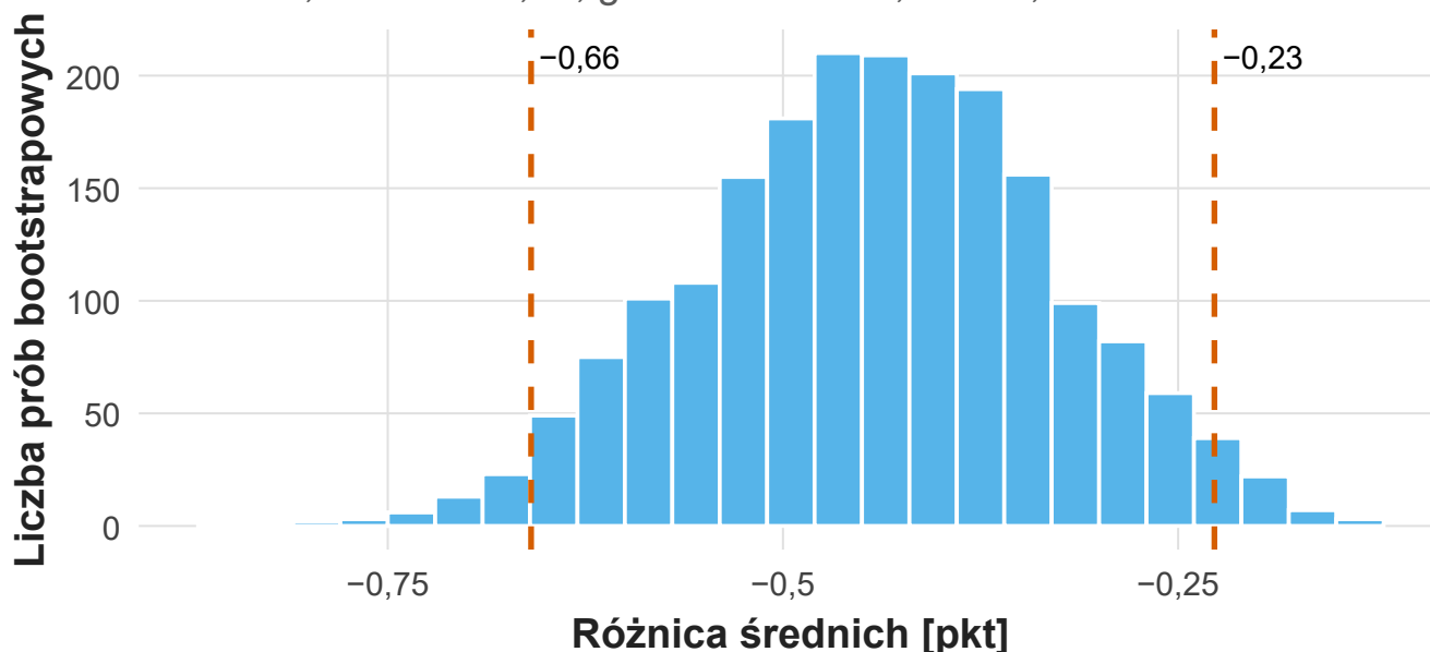
Rysunek 1: Tor bootstrapu w pierwszej analizie S02: 1999 różnic średnich z losowania osób ze zwracaniem w każdej grupie. Oś pozioma: różnica w punktach indeksu; linie przerywane oznaczają granice 95%, -0,66 i -0,23 .
