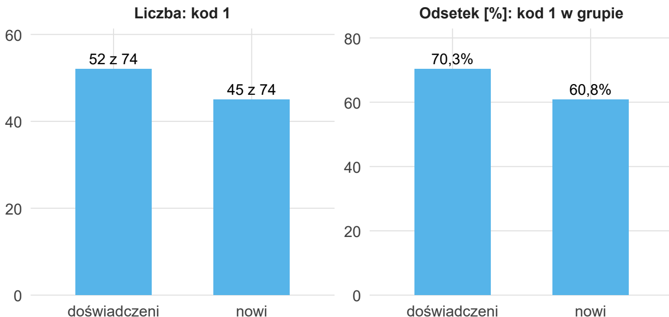
Rysunek 5: Kod 1 (znaleziony dokument) w grupach S02. Lewy panel: liczba osób z kodem 1; prawy panel: odsetek w grupie, 70,3% (52 z 74) u doświadczonych i 60,8% (45 z 74) u nowych.
