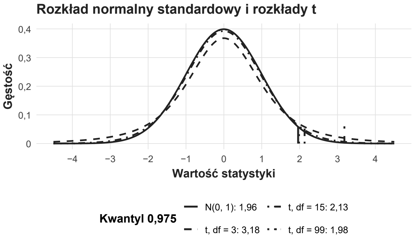
Rysunek 9: Rozkład normalny standardowy i rozkłady t. Oś pozioma: wartość statystyki od -4,5 do 4,5 ; oś pionowa: gęstość. Wszystkie krzywe są symetryczne wokół zera. Krzywa t z 3 stopniami swobody ma najniższy szczyt i najgrubsze ogony, a jej kwantyl 0,975 wynosi 3,18; krzywe t z 15 i 99 stopniami mają kwantyle 2,13 i 1,98, a rozkład normalny 1,96. Krótkie kreski przy osi oznaczają położenie kwantyli.
