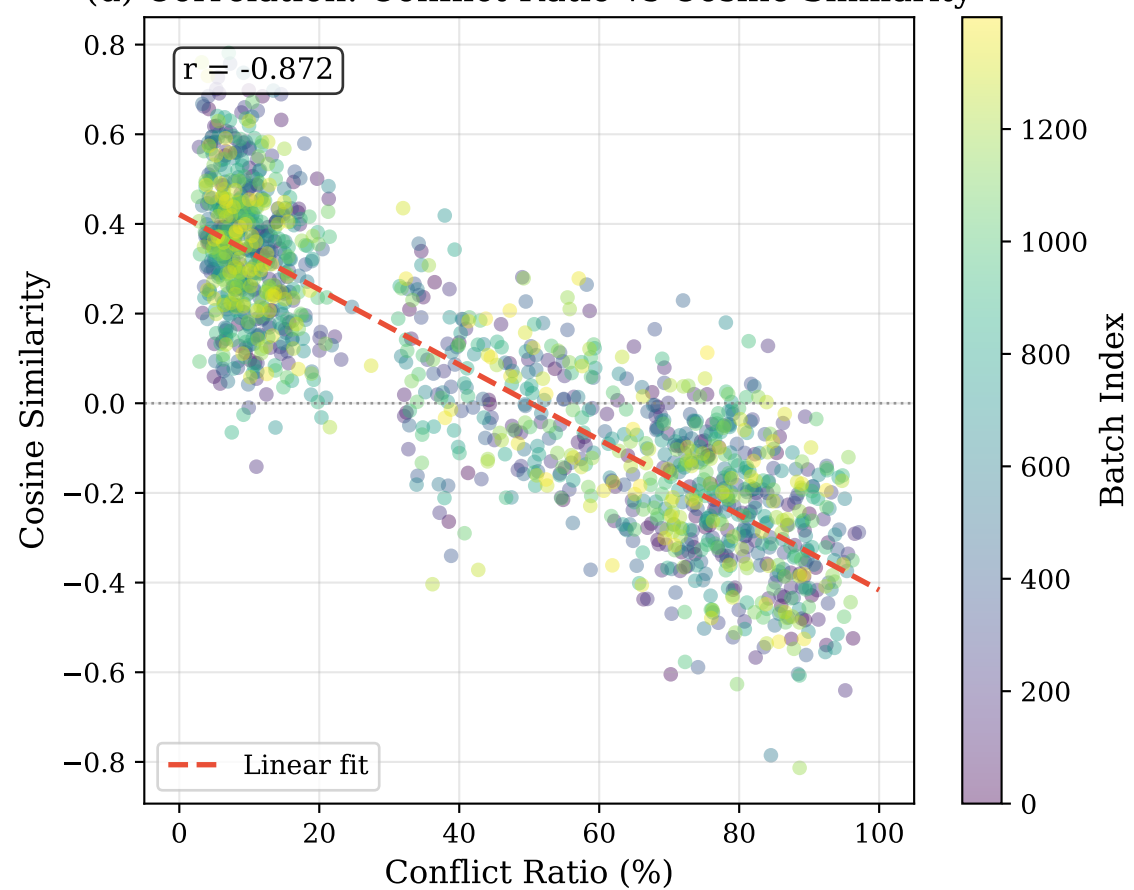
(d) Correlation: Conflict Ratio vs Cosine Similarity
