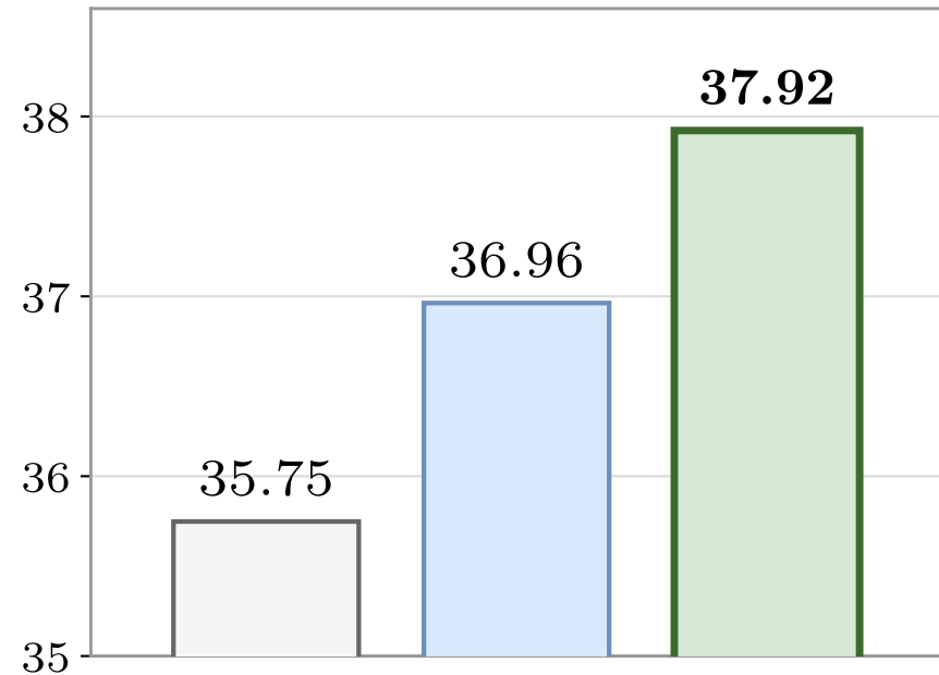
PSNR (dB) ↑
