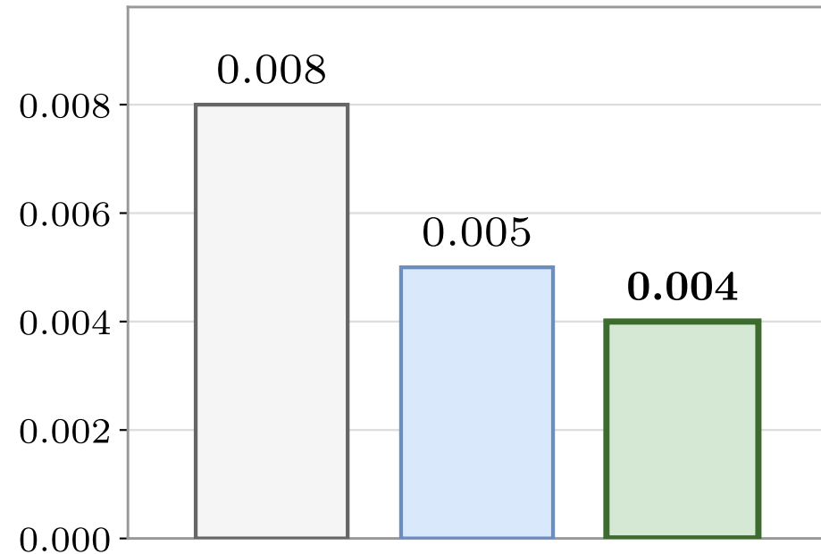
LPIPS ↓
