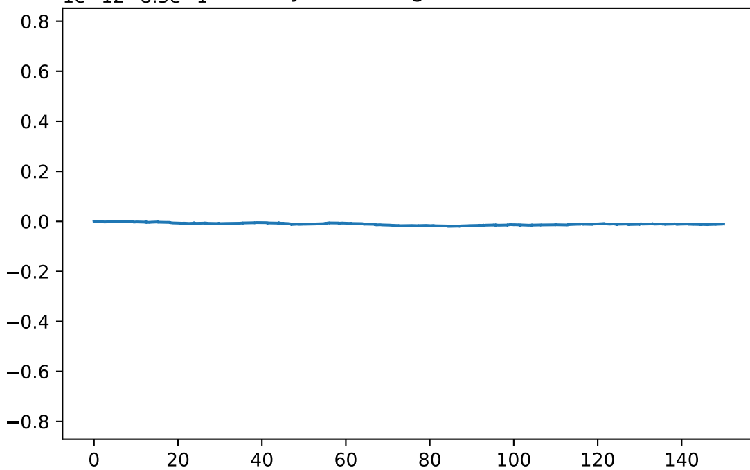
1e-12-8.5e-1 Velocity-Verlet Angular Momentum
