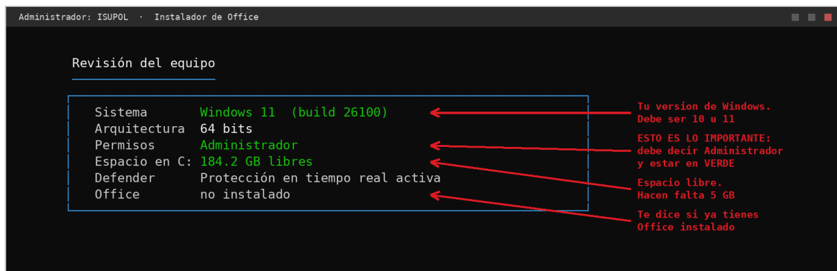
Figura 7. La tabla de revisión. Las flechas explican qué significa cada línea. La más importante es Permisos : tiene que decir «Administrador» y estar en verde.
