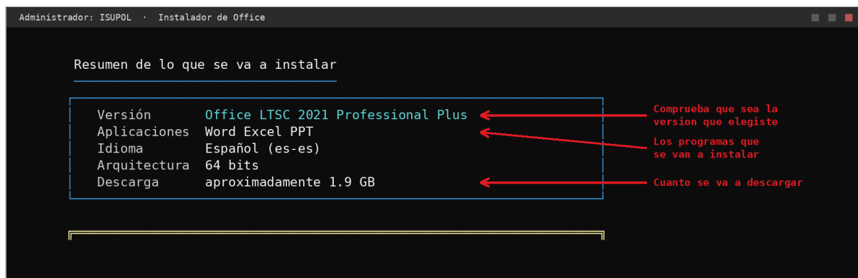
Figura 11. El resumen. Las flechas señalan las tres cosas que revisar: la versión, los programas que trae y cuánto se va a descargar.
