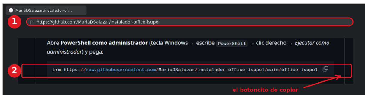
Figura 1. La página del instalador. Círculo 1: la barra de direcciones, ahí escribes la dirección. Círculo 2: el recuadro oscuro con el comando que copiaremos en el Paso D. La flecha señala el botoncito de copiar, que aparece al pasar el mouse por encima.
