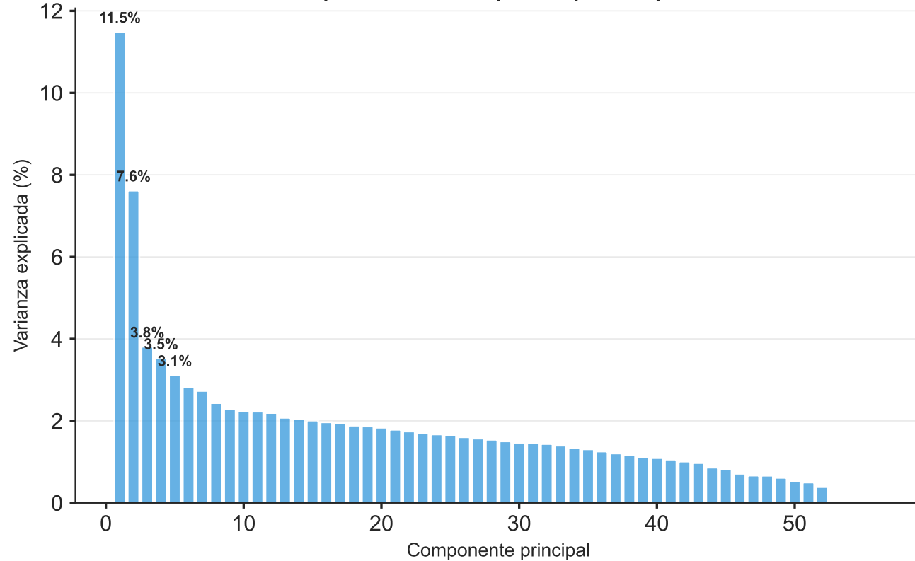
Scree plot – varianza explicada por componente
