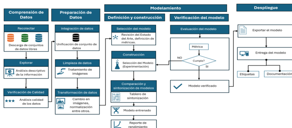
Ilustración 2 - Diagrama de Flujo de Datos general.
