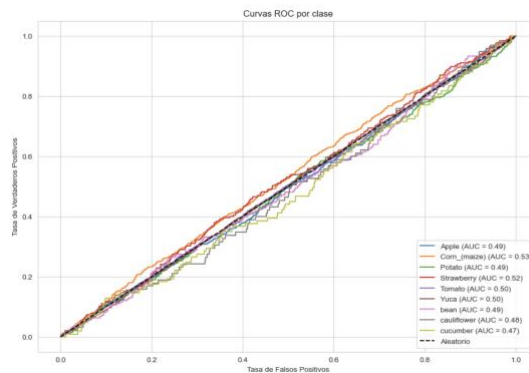
Ilustración 20 - Ejemplo de gráfica Curvas ROC por clase. Esta muestra corresponde al Modelo 1 (Versión conjunto de datos final)
