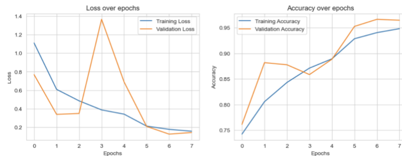
Ilustración 17 - Ejemplo gráficas de pérdida (loss) y precisión (accuracy). Esta gráfica corresponde al Modelo 1 (Versión conjunto de datos final)
