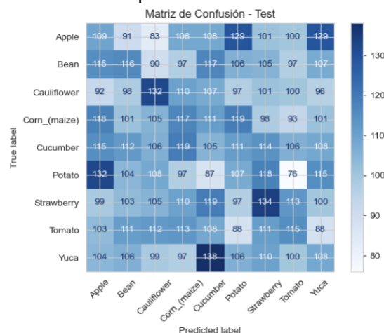
Ilustración 18 - Ejemplo matriz de confusión. Esta gráfica corresponde al Modelo 1 (Versión conjunto de datos final - Balanceado)
