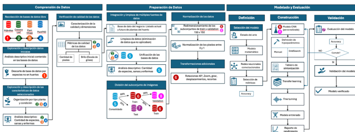
Ilustración Error! No text of specified style in document. 21 - Flujo de datos detallado (Comprensión, preparación de datos, modelado y evaluación) Fuente: Elaboración Propia
