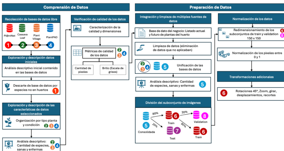
Ilustración 15 - Flujo de Datos (Comprensión y preparación de datos)
