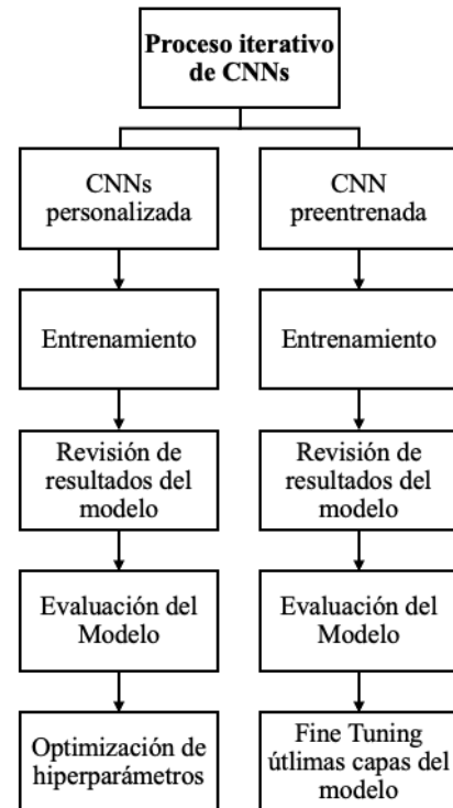
Ilustración 16 - Proceso iterativo de construcción de redes neuronales convolucionales
