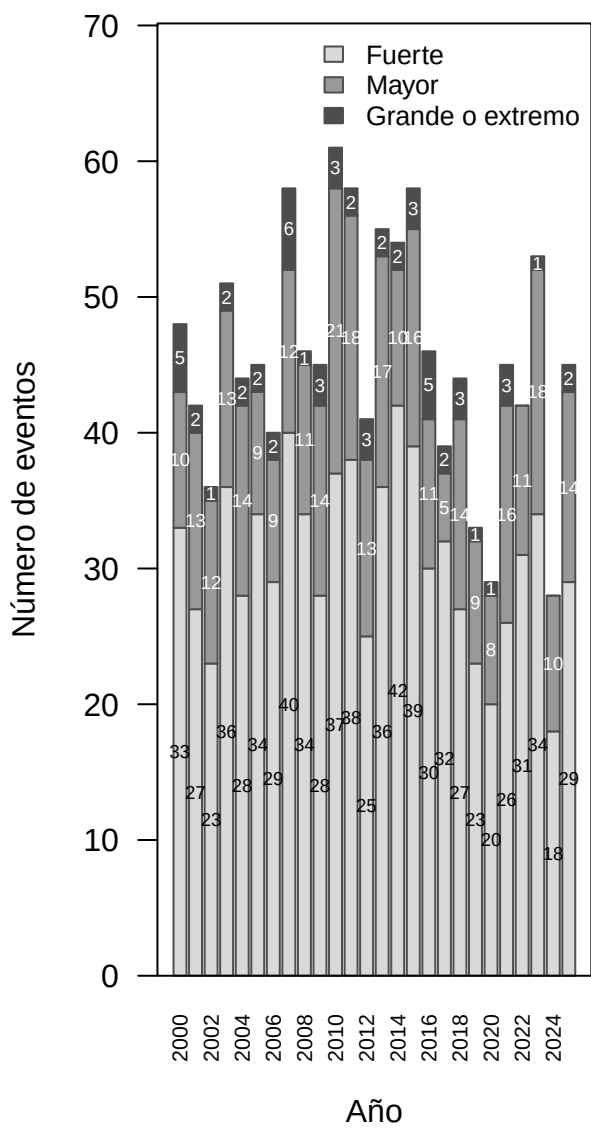
Eventos anuales por magnitud_ca
