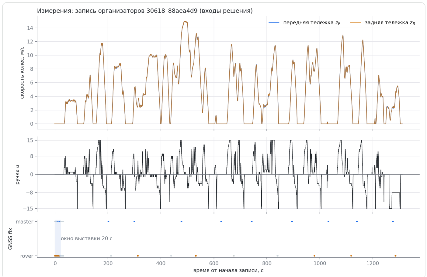
Рис. 1. Входы решения на записи организаторов 30618_88aea4d9.
