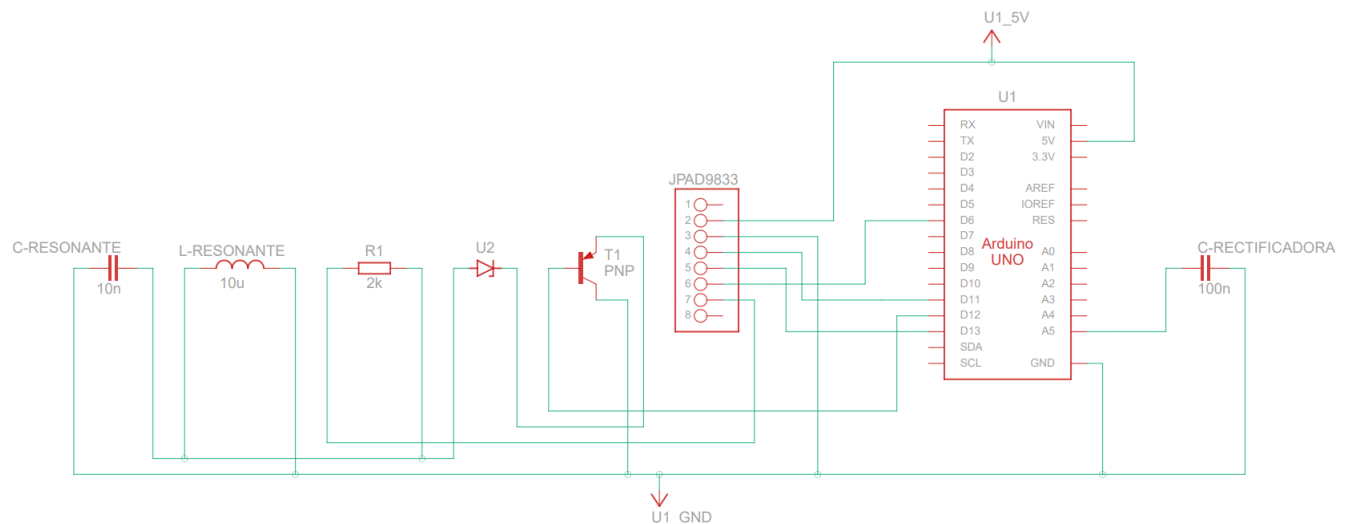
Figura 3.13: circuito donde se explica claramente la conexión del arduino
