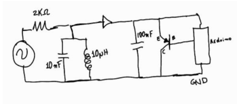
Figura 3.3: circuito dibujado a mano alzada
