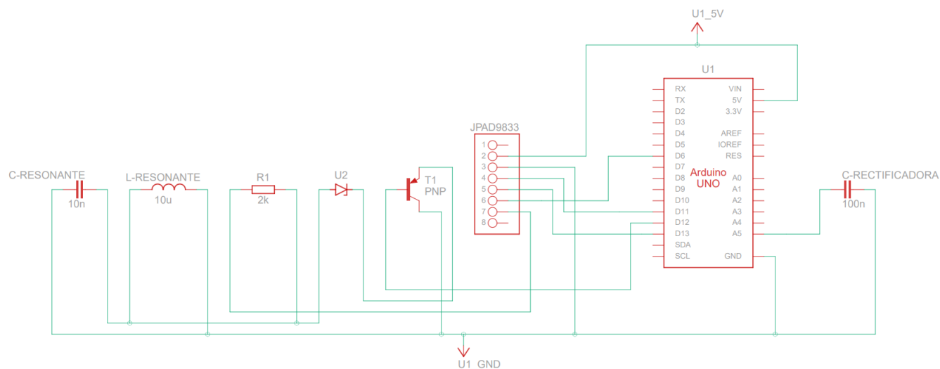
Figura 3.4: circuito donde se explica claramente la conexión del arduino
