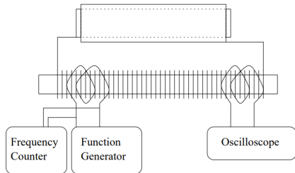
Circuito resonante por inducción (MIT, Junior Physics Lab).
