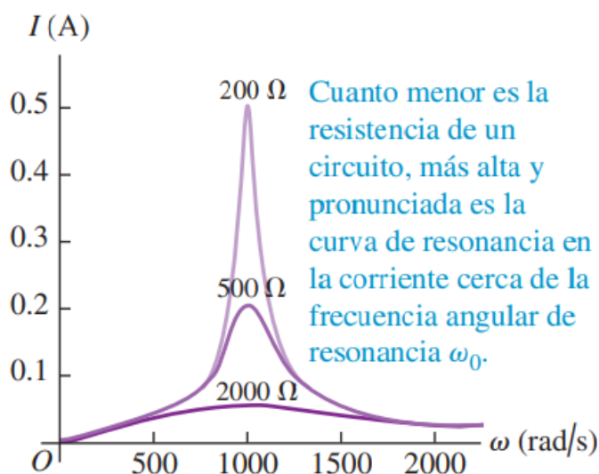
Figura 3.1: Comportamiento del factor Q según la resistencia en el circuito [19].
