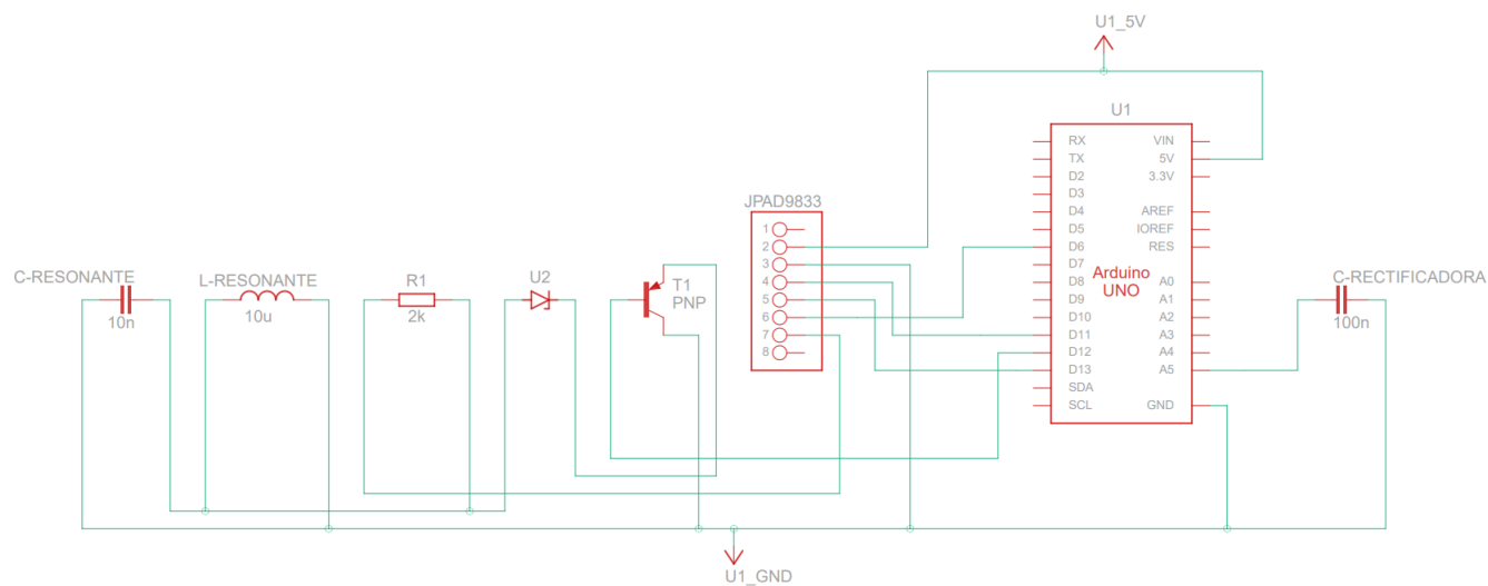
Figura 3.6: circuito donde se explica claramente la conexión del arduino
