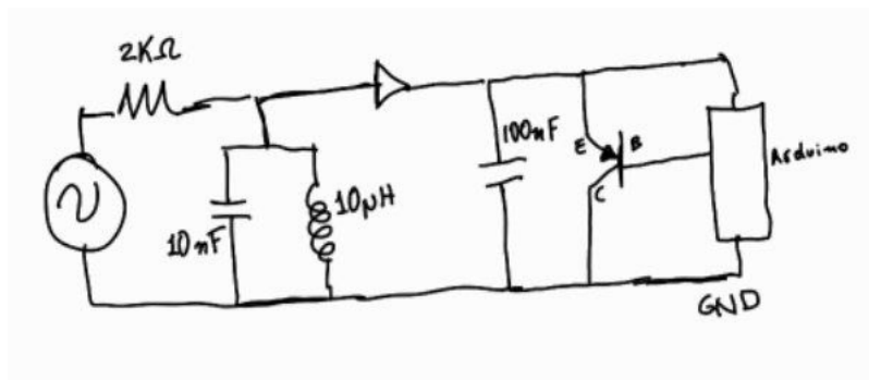
Figura 3.5: circuito dibujado a mano alzada
