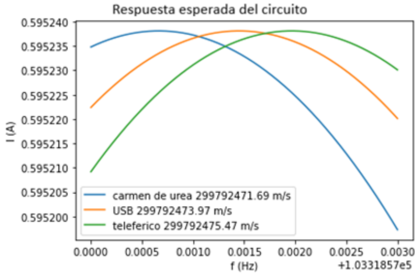
Figura 3.3: Curvas I(f) para las tres locaciones.
