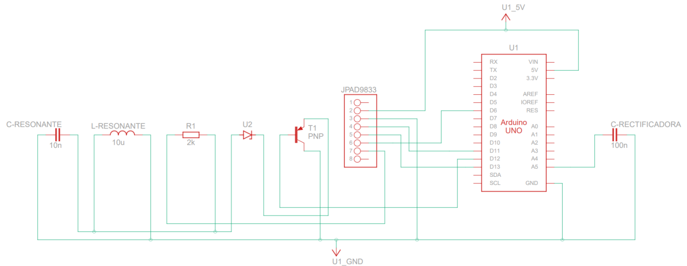
Figura 3.17: circuito donde se explica claramente la conexión del arduino
