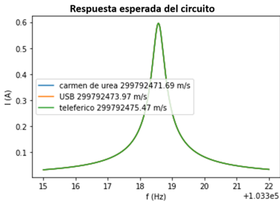
Figura 3.4: Detalle de la curva I(f) .
