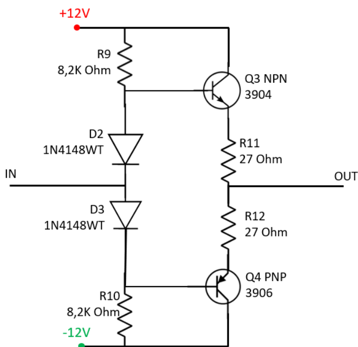
Figura 3.16: Esquemático de la etapa amplificadora de potencia del amplificador 1 en el experimento conectado en serie.
