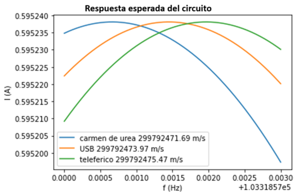
Figura 3.3: Curvas I(f) para las tres locaciones.
