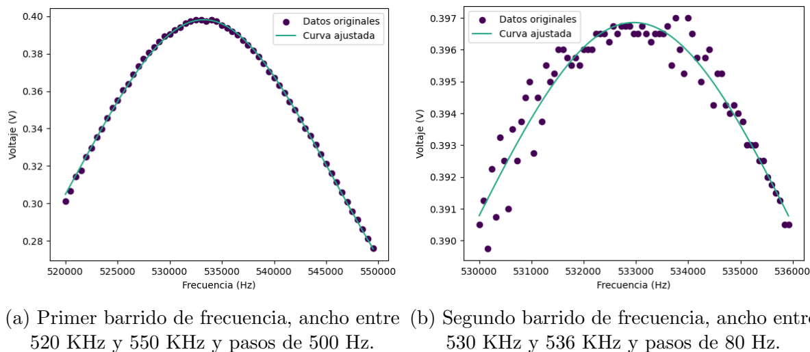
Figura 3.16: Gráficas de los barridos de frecuencia con mejores resultados del experimento en paralelo, incluye los datos originales y la curva ajustada.
