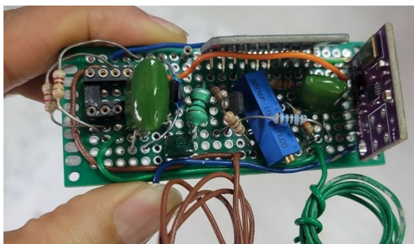
(a) Prototipo elaborado con placa perforada.
