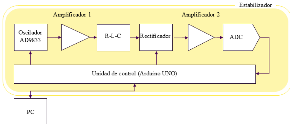
Figura 3.6: Módulos del experimento.
