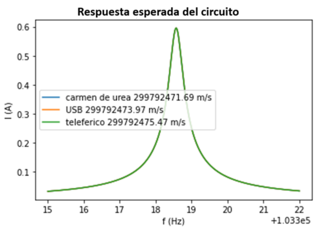
Figura 3.4: Detalle de la curva I(f) .
