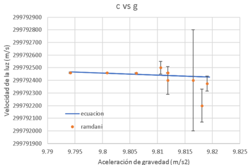
Figura 1.3: Datos de velocidad de la luz vs gravedad incluidos en la tabla 1.2 superpuestos a la línea predicha por HCC en la ecuación 1.42
