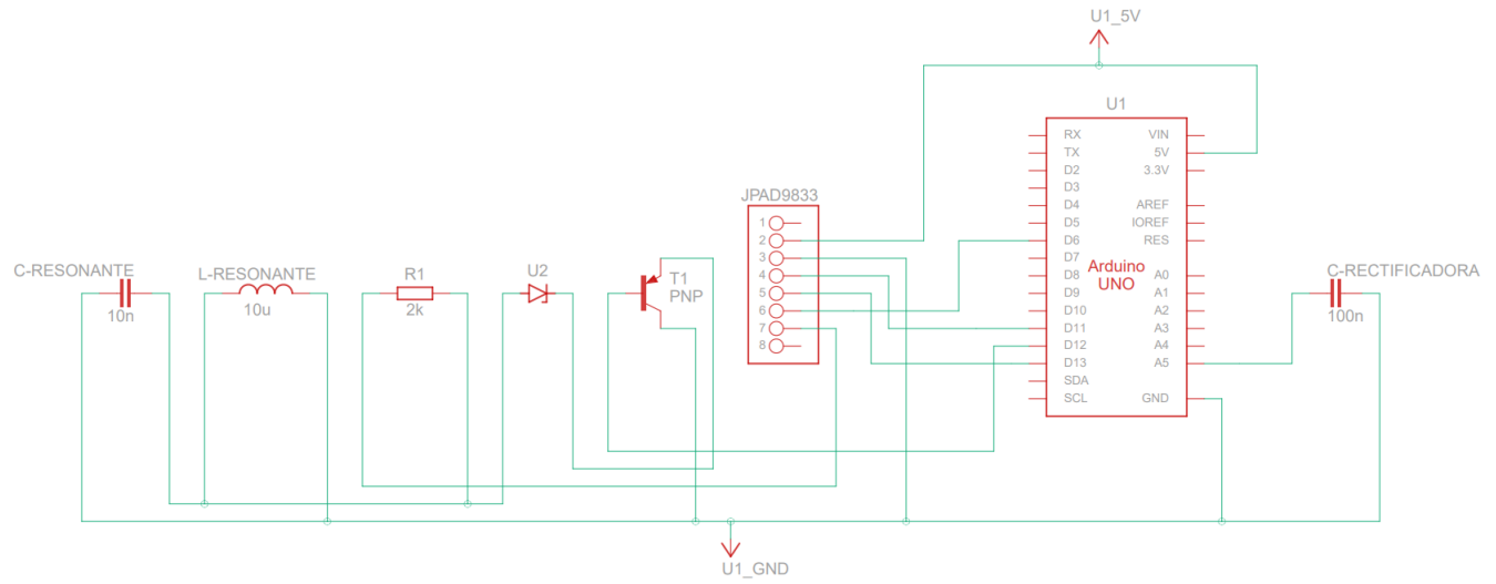
Figura 3.18: circuito donde se explica claramente la conexión del arduino
