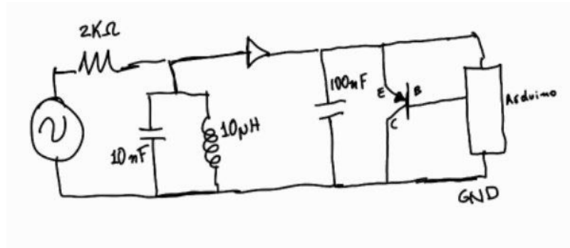
Figura 3.8: circuito dibujado a mano alzada
