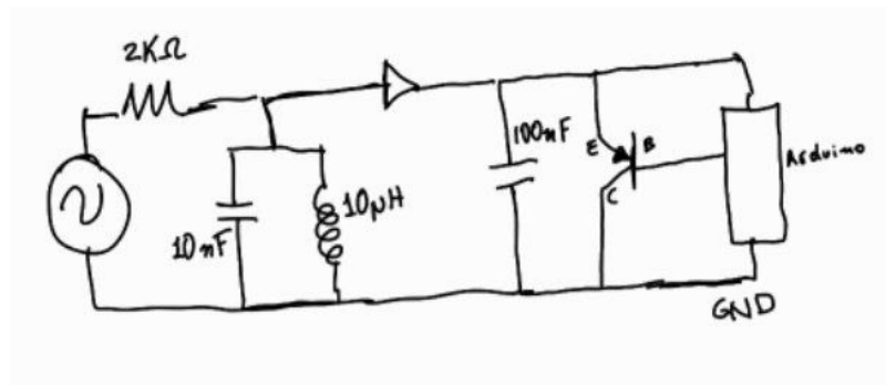
Figura 3.10: circuito dibujado a mano alzada
