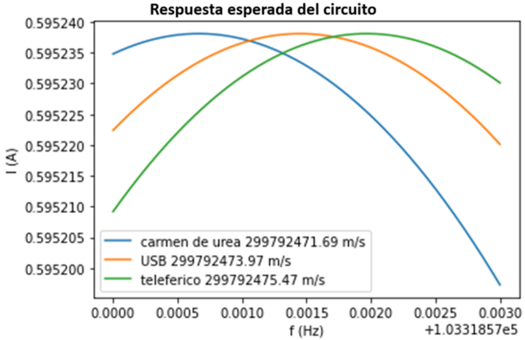
Figura 3.3: Curvas I(f) para las tres locaciones.
