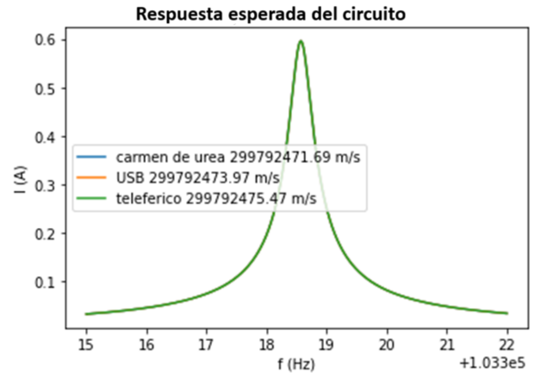
Figura 3.4: Detalle de la curva I(f) .
