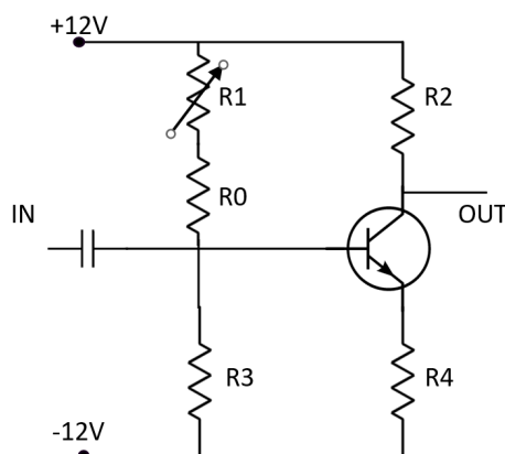
Figura 3.7: Esquemático de la etapa amplificadora de voltaje perteneciente al Amplificador 1 del módulo generador.
