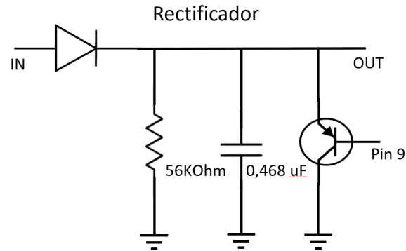
Figura 3.8: Esquemático del rectificador” perteneciente al módulo de lectura.
