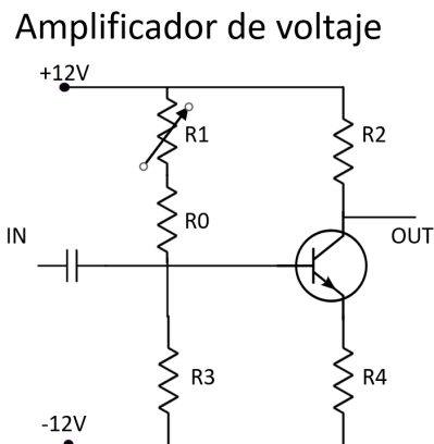
Figura 3.7: Esquemático de la etapa amplificadora de voltaje perteneciente al Amplificador 1 del módulo generador.
