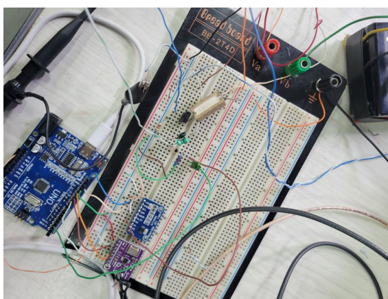
Figura 3.14: Foto de experimento RLC en paralelo.
