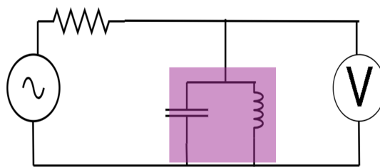
Figura 3.5: Esquema básico de circuito RLC en paralelo.
