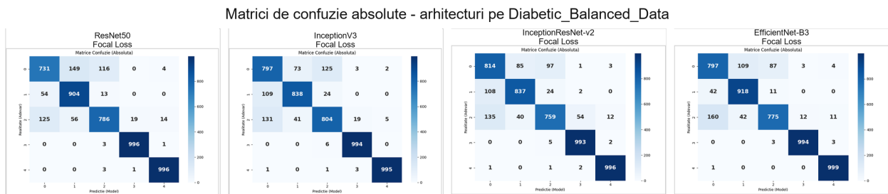
Figura 6.2: Matrici de confuzie absolute pentru arhitecturile comparate pe Diabetic_Balanced_Data.
