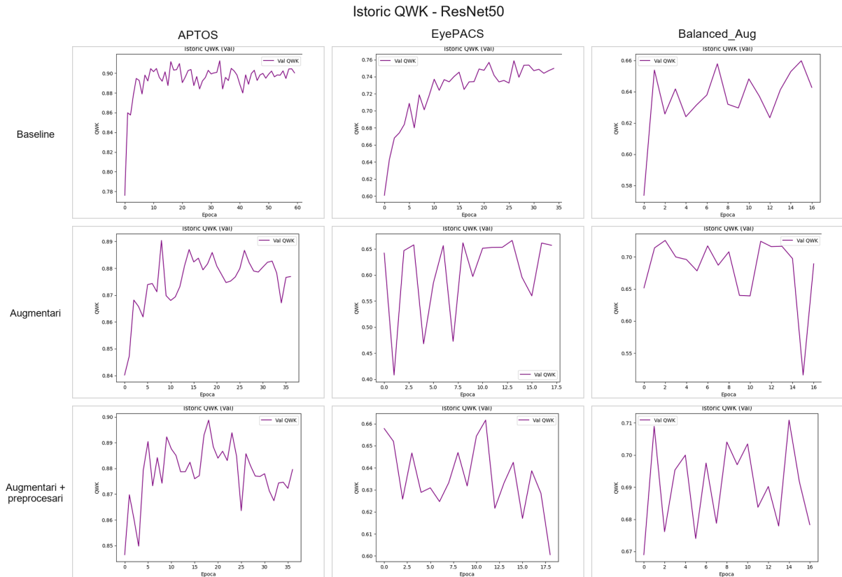
Figura 6.7: Istoricul scorului QWK pentru ResNet50 pe cele 9 variante de experimente.
