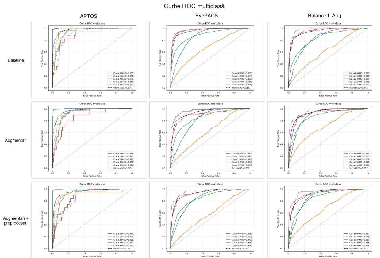
Figura 6.10: Curbele ROC multclasă pentru cele nouă experimente principale din experiments.ipynb .
