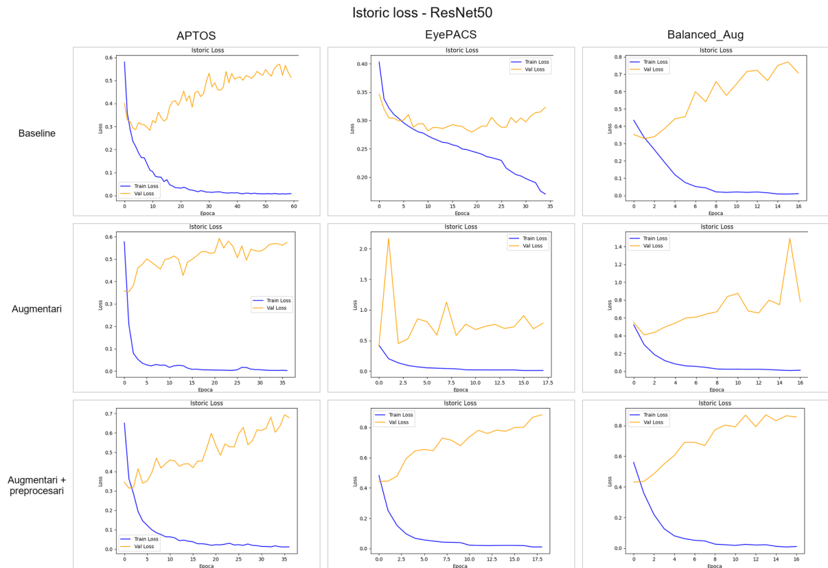
Figura 6.5: Istoricul loss-ului pentru ResNet50 pe APTOS, EyePACS și Balanced_Aug.
