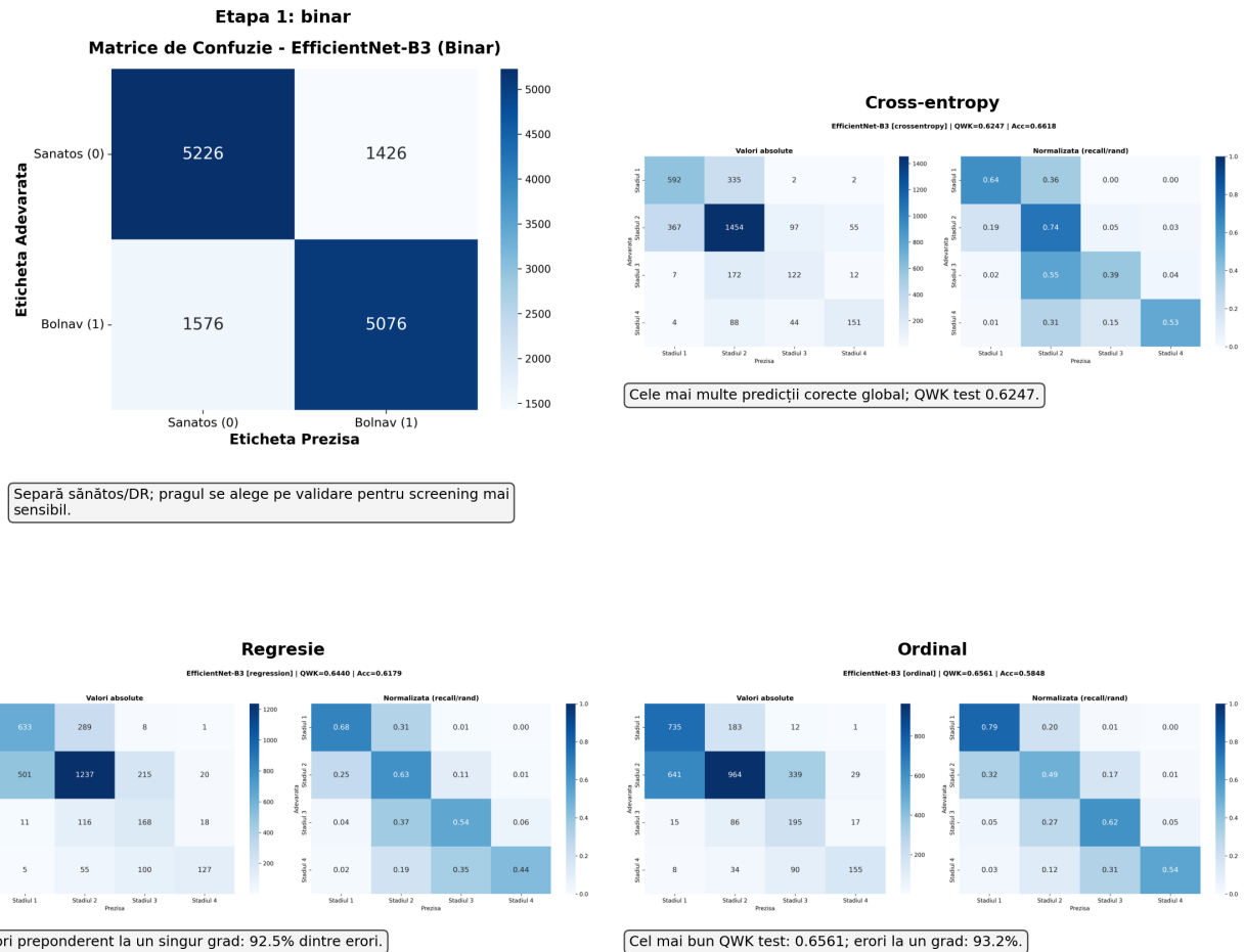
Figura 6.12: Matrici de confuzie combinate pentru etapa binară și pentru cele trei variante multclasă. Comentariile evidențiază diferența dintre acuratețe globală și respectarea ordinii clinice a claselor.
