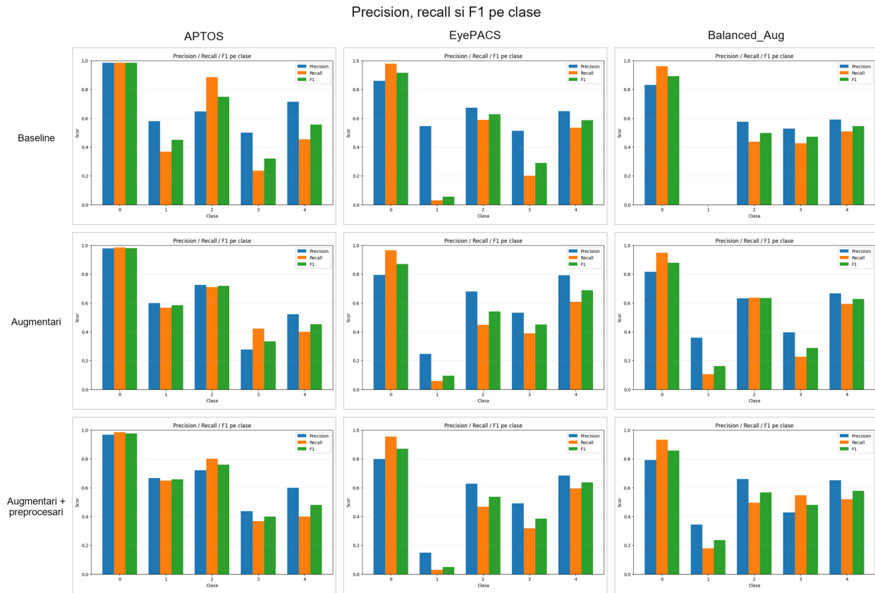
Figura 6.8: Precision, recall și F1 pe clase pentru cele nouă experimente principale.
