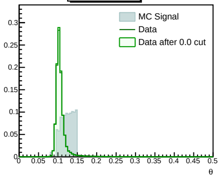
S19pos_mod
