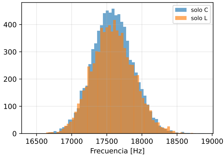
f_0 variando una reactancia
