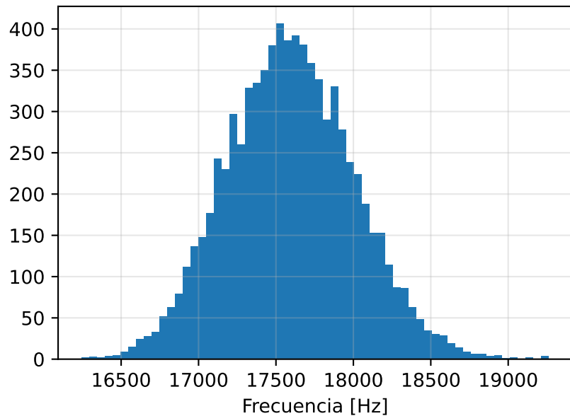
f_0 variando una reactancia
