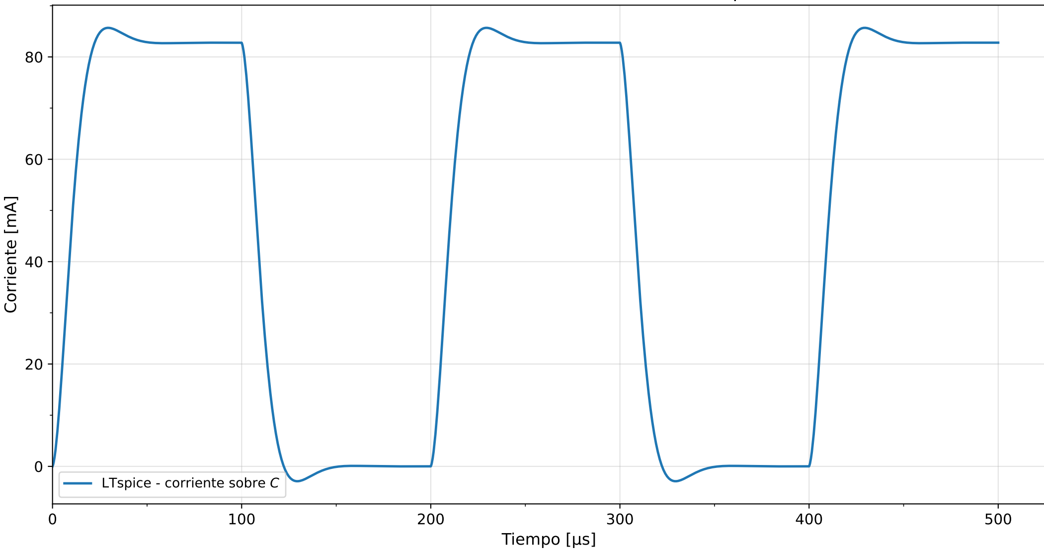
Transitorio 2.1 - corriente simulada sobre el capacitor
