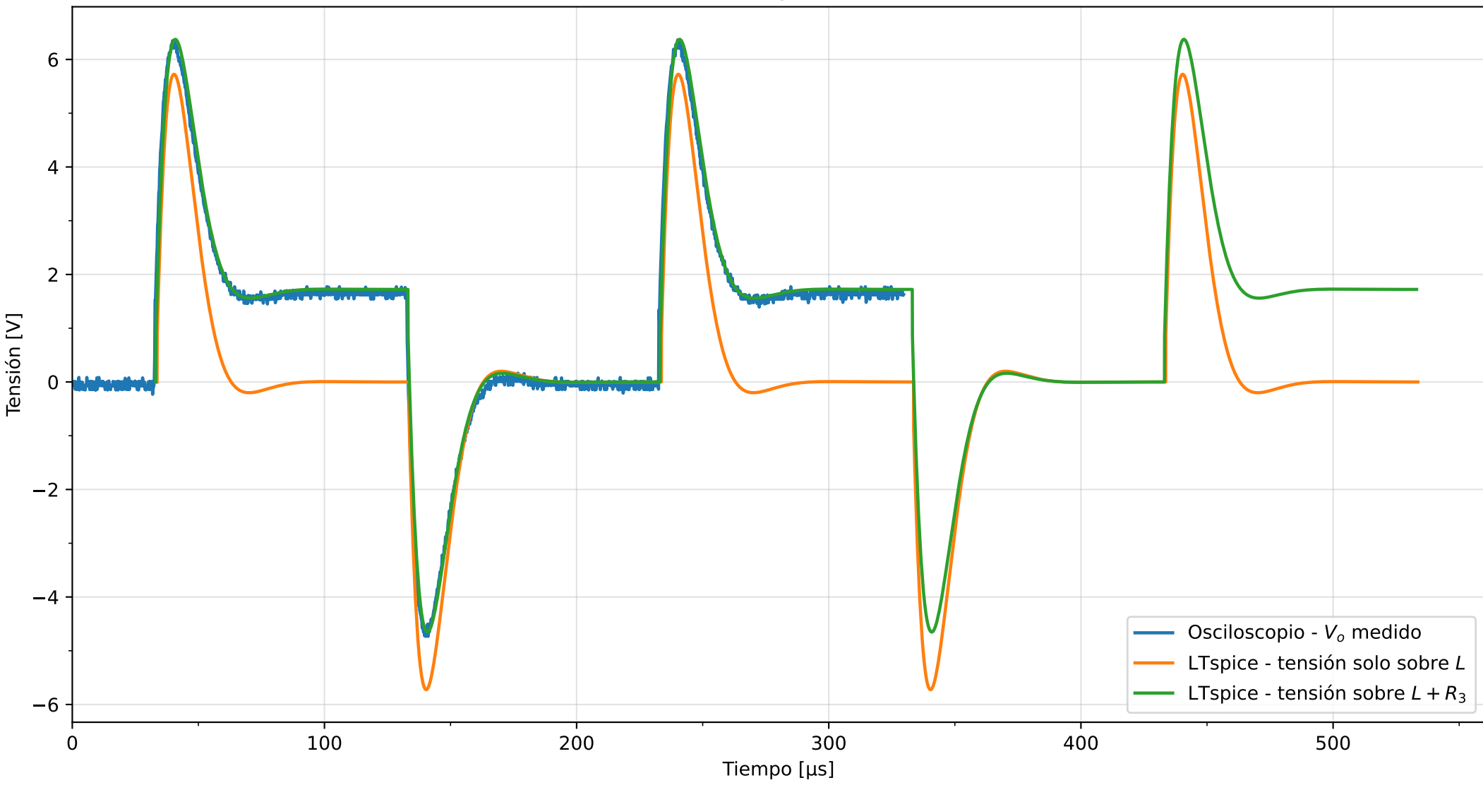
Transitorio 2.1 - medición y simulaciones de tensión
