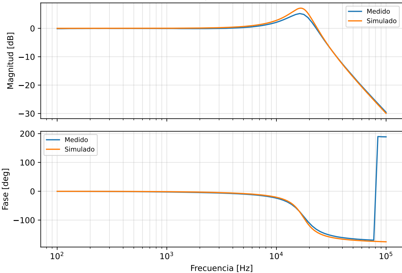
Circuito 2: respuesta en frecuencia
