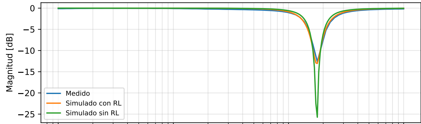
Circuito 5: efecto de resistencia serie del inductor
