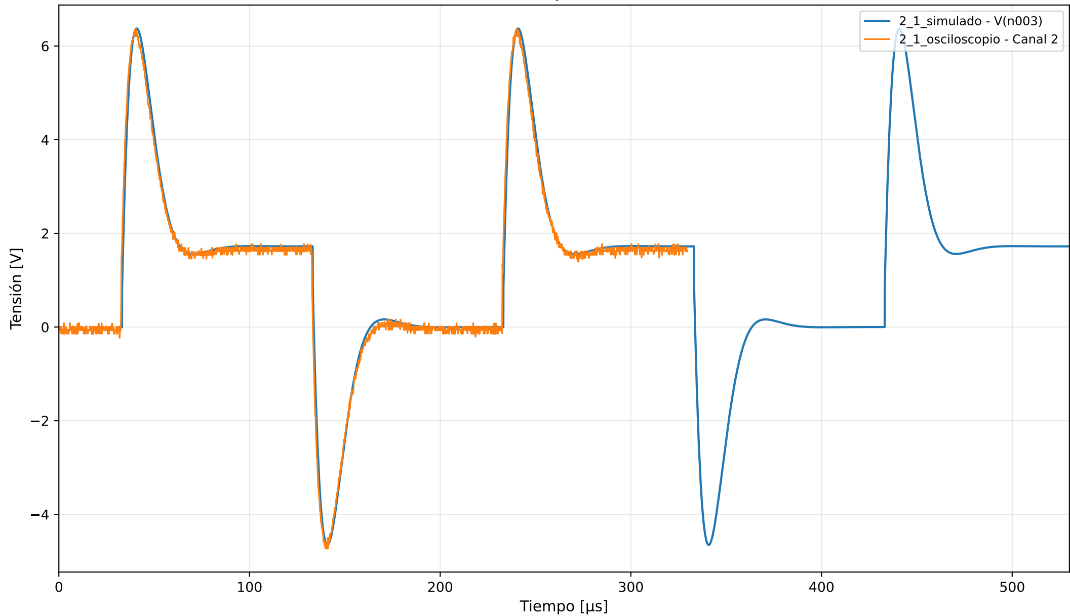
Transitorio 2.1: simulación y medición alineadas en fase
