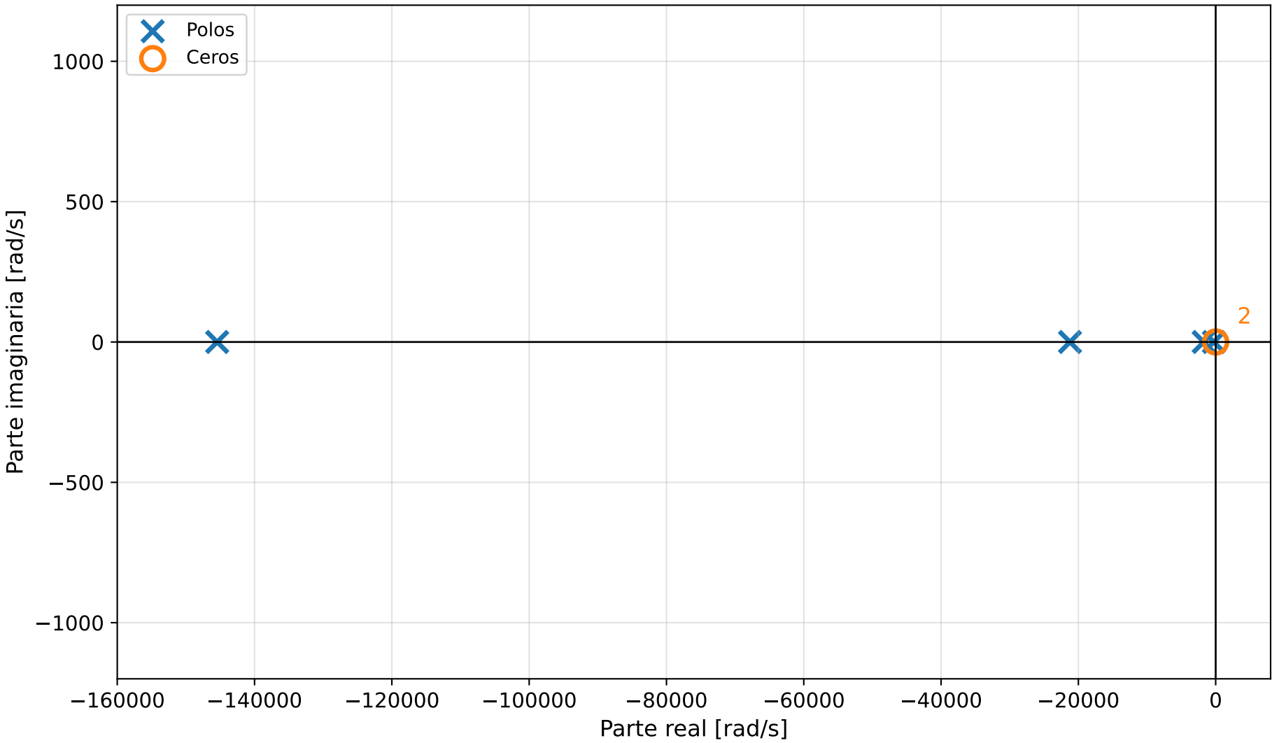
Filtro final - diagrama de polos y ceros
