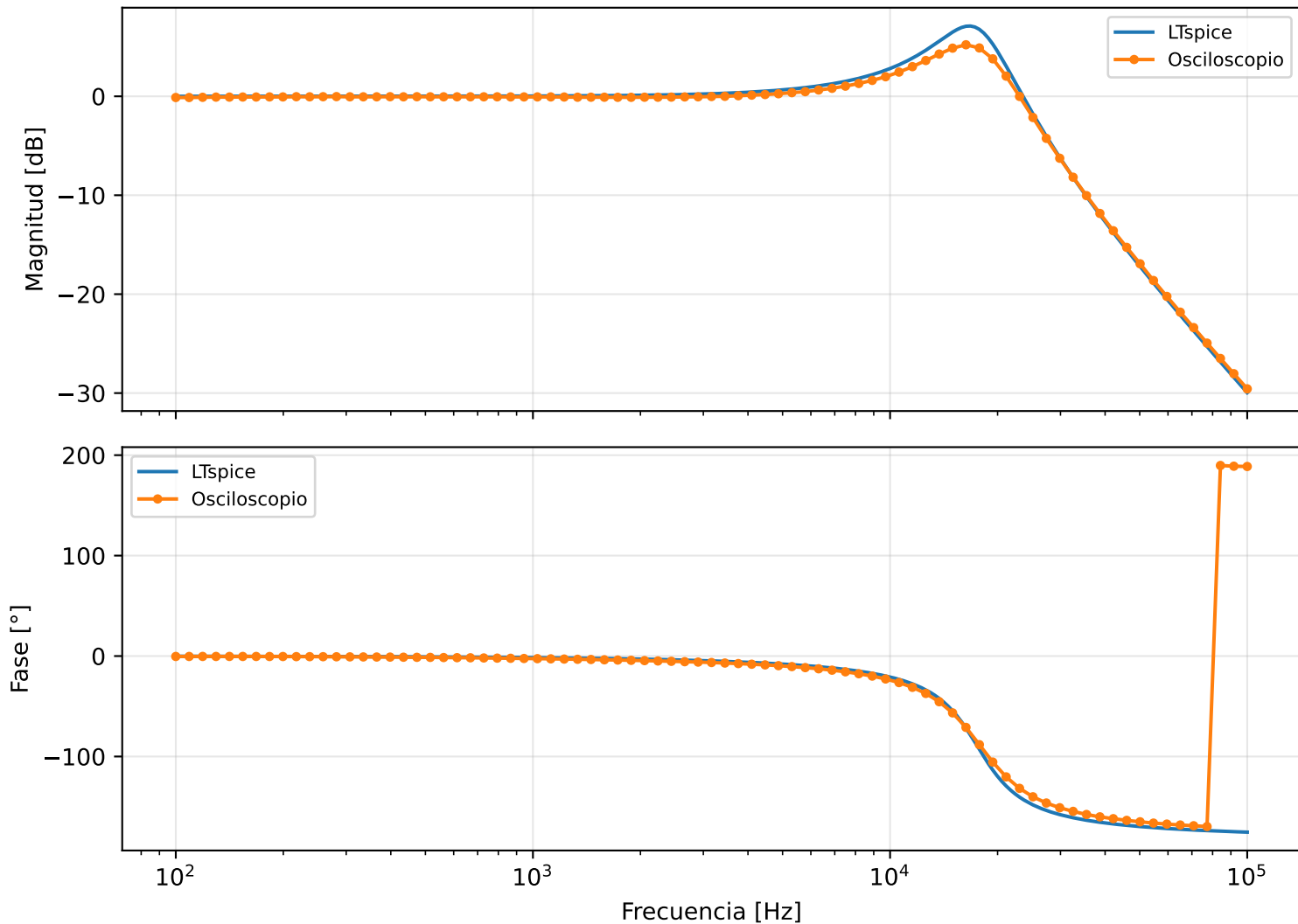
Circuito 2 - pasabajos
