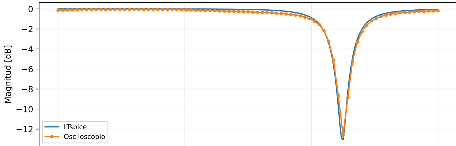
Circuito 5 - rechazo de banda
