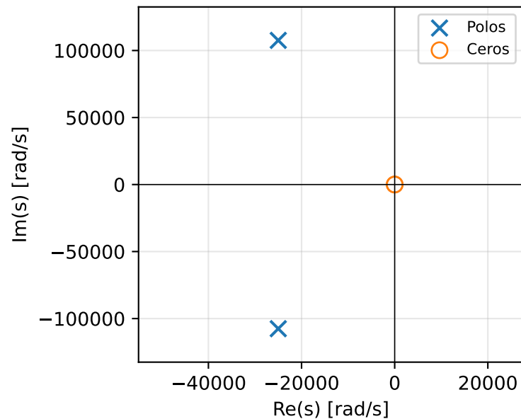
Circuito 5
