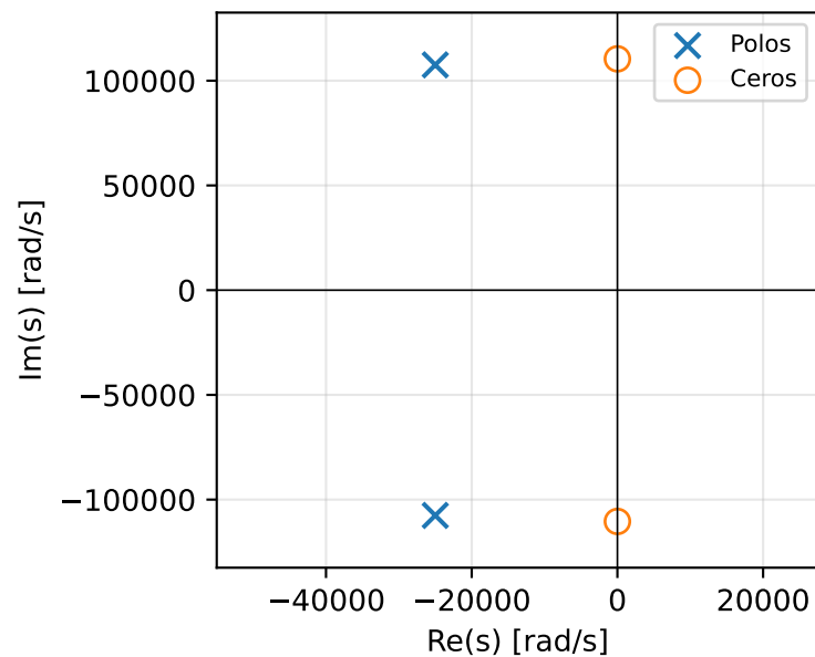
Circuito 5
